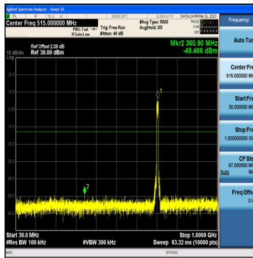
Band12-10MHz-QPSK-23130-50RB#0-Range1:30~1000MHz
