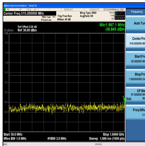
Band25-20MHz-QPSK-26365-100RB#0-Range1:30~1000MHz
