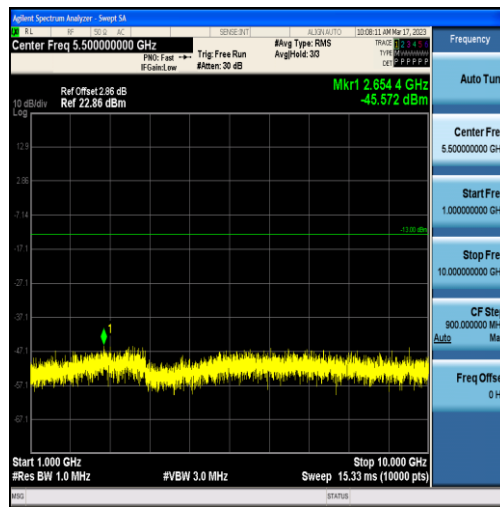
Band71-10MHz-QPSK-133297-50RB#0-Range2:1000~10000MHz
