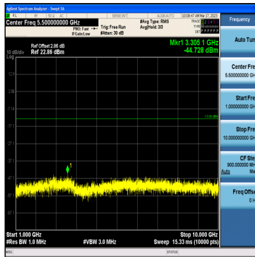
Band71-10MHz-QPSK-133422-50RB#0-Range2:1000~10000MHz
