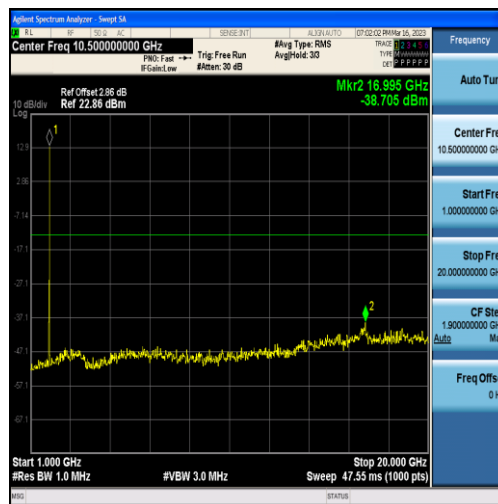
Band25-10MHz-QPSK-26640-50RB#0-Range2:1000~20000MHz
