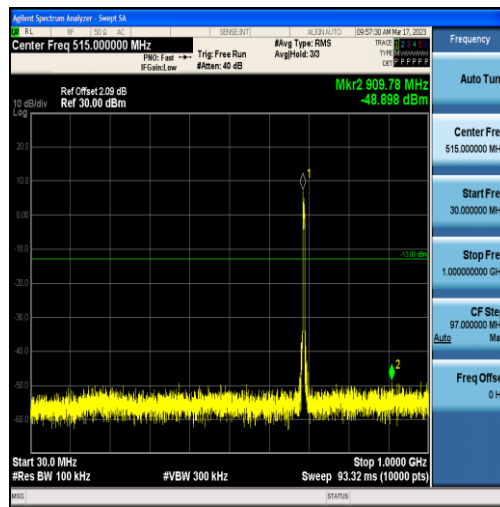
Band71-5MHz-QPSK-133447-25RB#0-Range1:30~1000MHz
