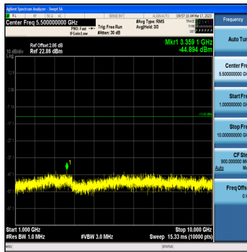
Band71-5MHz-QPSK-133297-25RB#0-Range2:1000~10000MHz
