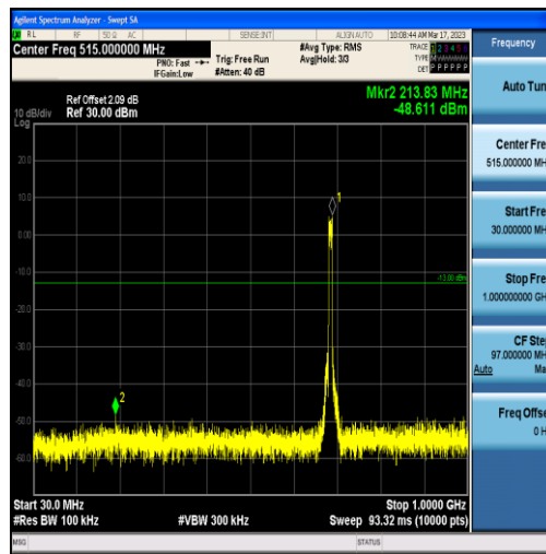
Band71-10MHz-QPSK-133422-50RB#0-Range1:30~1000MHz
