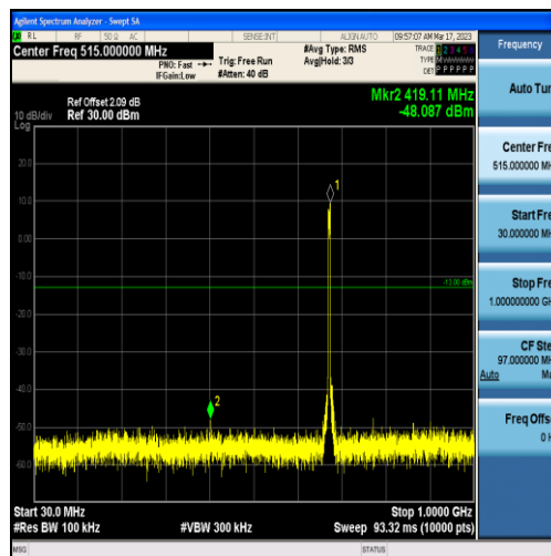
Band71-5MHz-QPSK-133297-25RB#0-Range1:30~1000MHz
