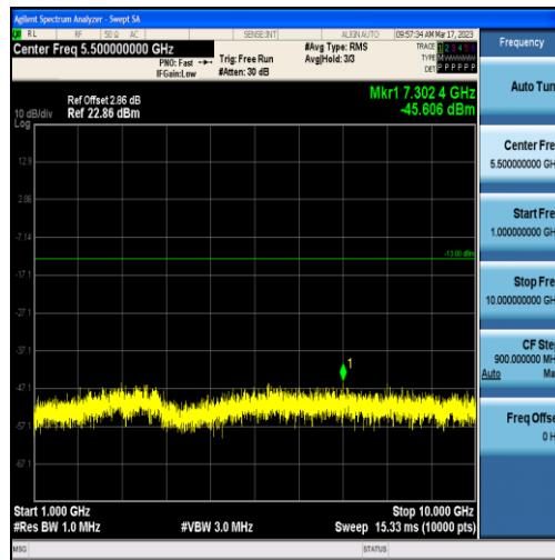
Band71-5MHz-QPSK-133447-25RB#0-Range2:1000~10000MHz
