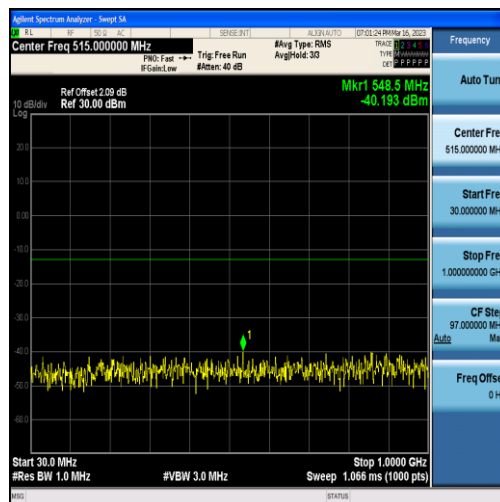
Band25-10MHz-QPSK-26365-50RB#0-Range1:30~1000MHz
