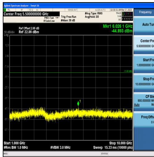
Band71-20MHz-QPSK-133297-100RB#0-Range2:1000~10000MHz
