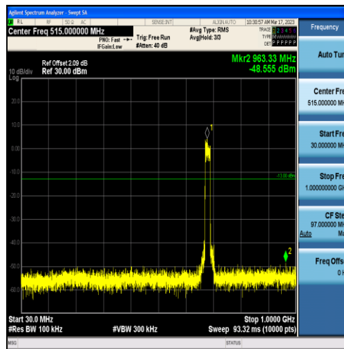
Band71-20MHz-QPSK-133372-100RB#0-Range1:30~1000MHz
