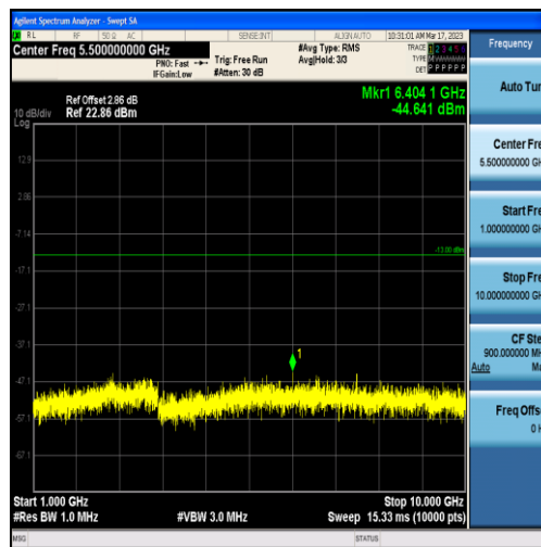
Band71-20MHz-QPSK-133372-100RB#0-Range2:1000~10000MHz
