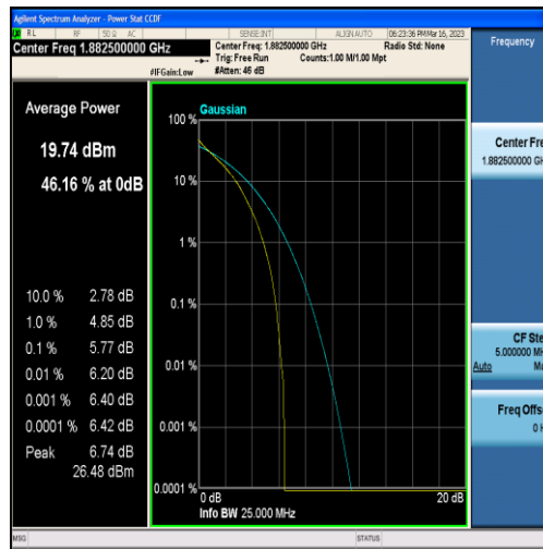
Band25-1.4MHz-QPSK-26365-6RB#0
