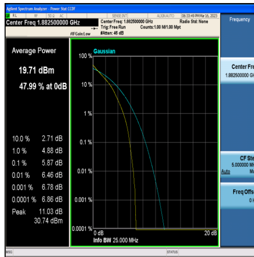
Band25-3MHz-QPSK-26365-15RB#0
