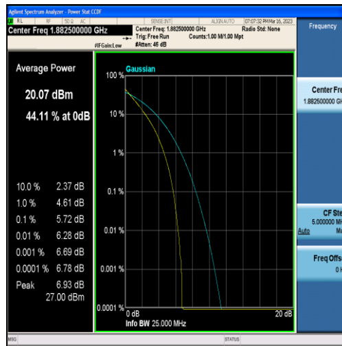
Band25-10MHz-QPSK-26365-50RB#0
