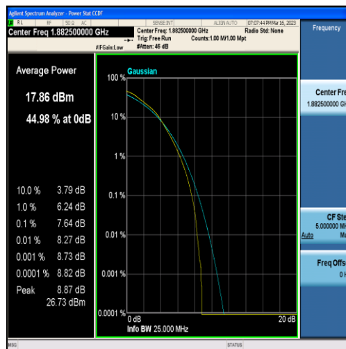
Band25-10MHz-16QAM-26365-50RB#0
