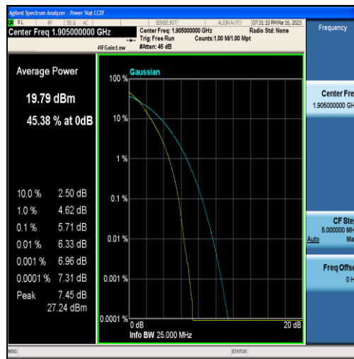
Band25-20MHz-QPSK-26590-100RB#0
