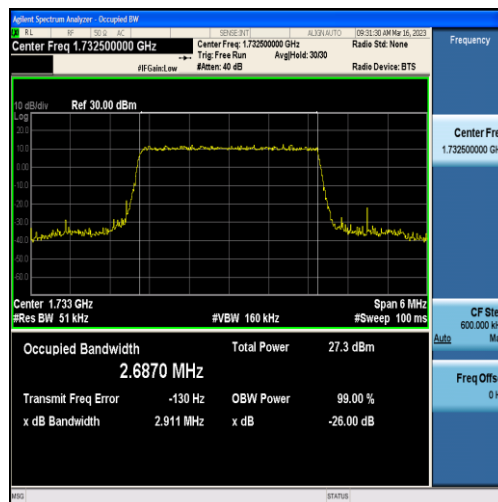
Band4-3MHz-QPSK-20175-15RB#0-2.6870
