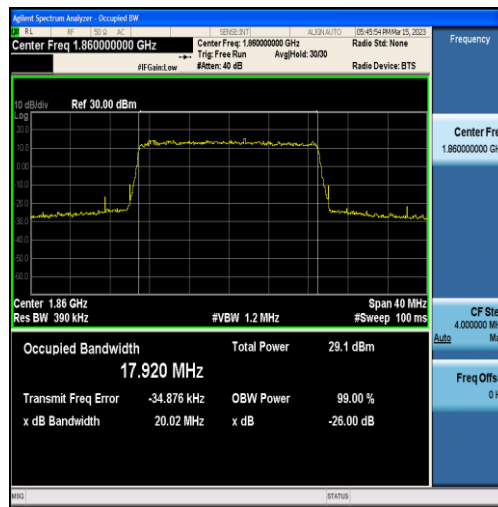
Band2-20MHz-QPSK-18700-100RB#0-17.920
