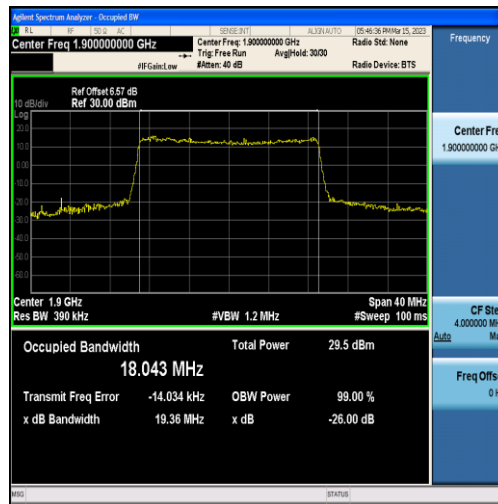
Band2-20MHz-QPSK-19100-100RB#0-18.043
