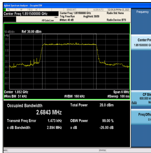
Band2-3MHz-QPSK-18615-15RB#0-2.6843
