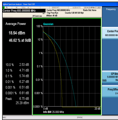
Band71-10MHz-QPSK-133422-50RB#0
