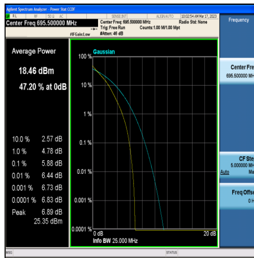
Band71-5MHz-QPSK-133447-25RB#0
