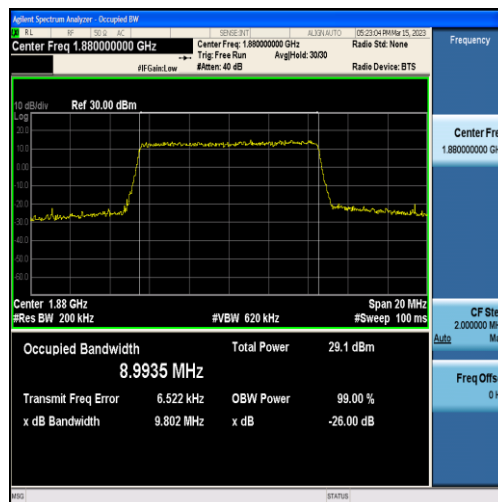
Band2-10MHz-QPSK-18900-50RB#0-8.9935
