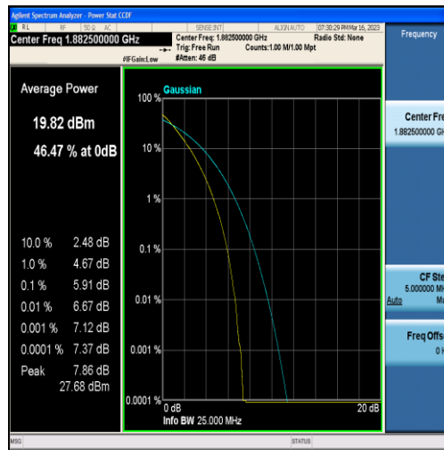
Band25-20MHz-QPSK-26365-100RB#0
