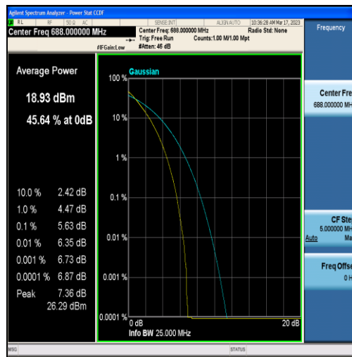
Band71-20MHz-QPSK-133372-100RB#0
