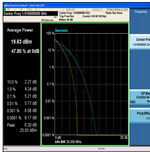
Band25-10MHz-QPSK-26640-50RB#0
