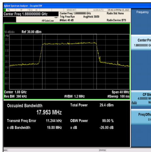
Band2-20MHz-QPSK-18900-100RB#0-17.953
