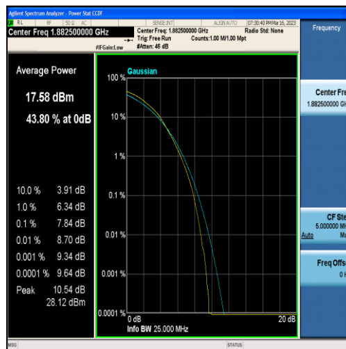
Band25-20MHz-16QAM-26365-100RB#0
