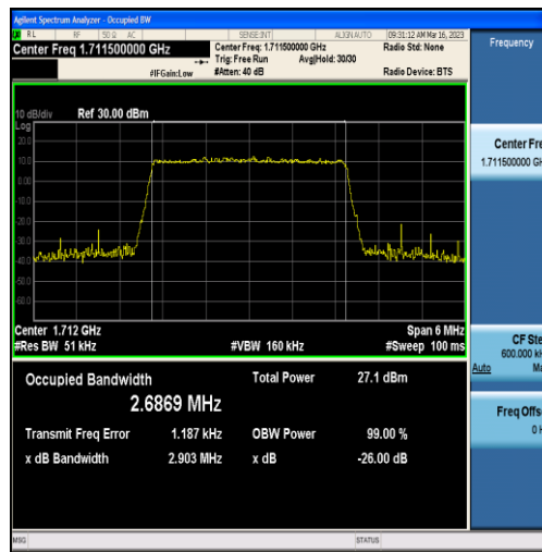
Band4-3MHz-QPSK-19965-15RB#0-2.6869
