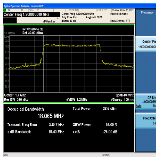
Band2-20MHz-16QAM-19100-100RB#0-18.065
