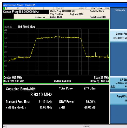
Band71-10MHz-QPSK-133172-50RB#0-8.9310
