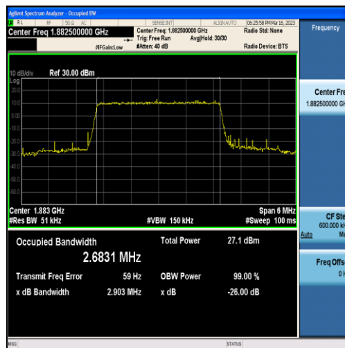
Band25-3MHz-16QAM-26365-15RB#0-2.6831
