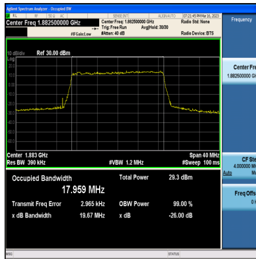
Band25-20MHz-QPSK-26365-100RB#0-17.959
