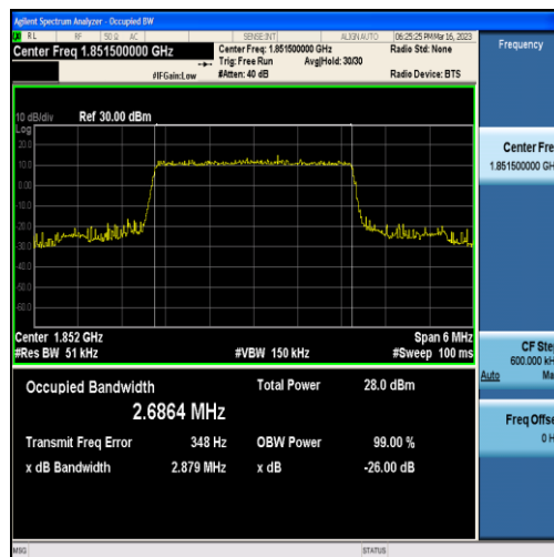
Band25-3MHz-QPSK-26055-15RB#0-2.6864
