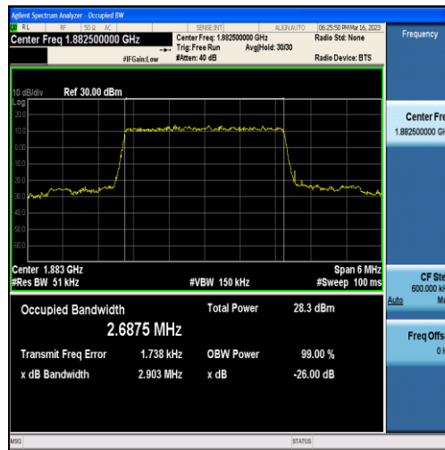
Band25-3MHz-QPSK-26365-15RB#0-2.6875
