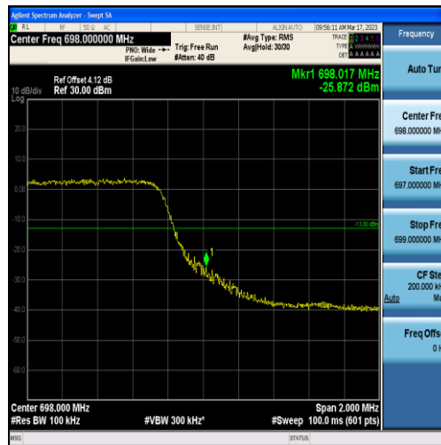
Band71-5MHz-QPSK-133447-25RB#0
