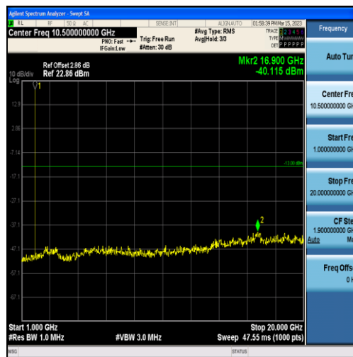
Band2-1.4MHz-QPSK-19193-6RB#0-Range2:1000~20000MHz
