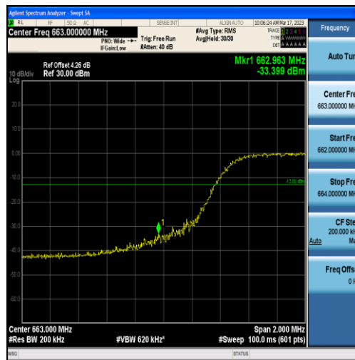
Band71-10MHz-QPSK-133172-50RB#0
