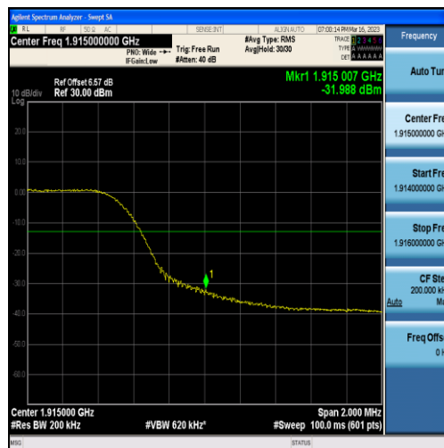
Band25-10MHz-QPSK-26640-50RB#0
