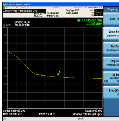
Band25-20MHz-QPSK-26590-100RB#0
