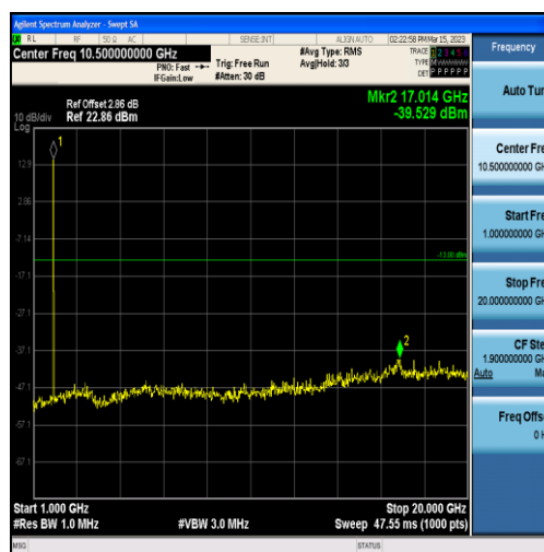
Band2-5MHz-16QAM-18900-25RB#0-Range2:1000~20000MHz
