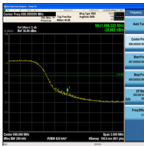
Band71-10MHz-QPSK-133422-50RB#0
