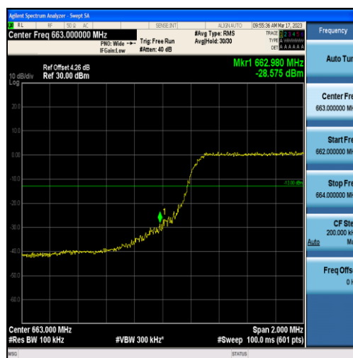
Band71-5MHz-QPSK-133147-25RB#0
