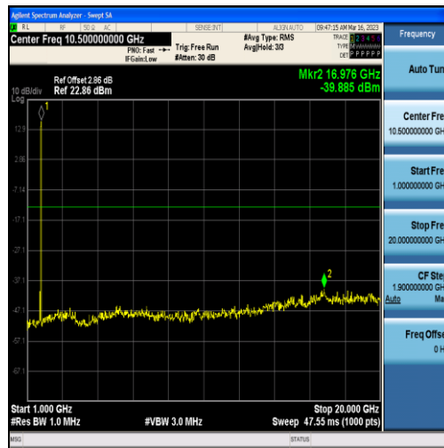
Band4-5MHz-QPSK-20375-25RB#0-Range2:1000~20000MHz
