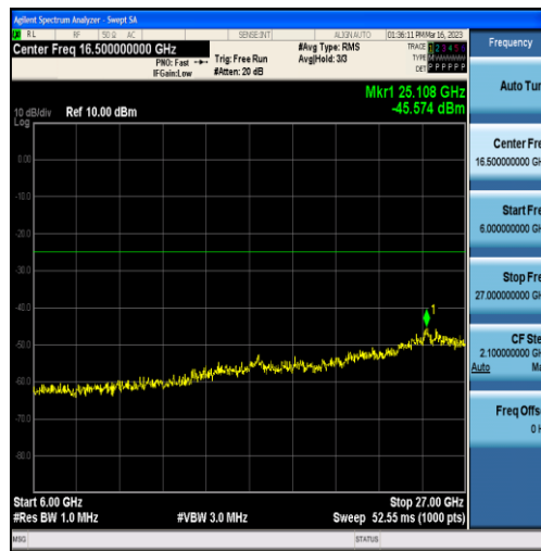
Band7-5MHz-QPSK-20775-25RB#0-Range3:6000~27000MHz
