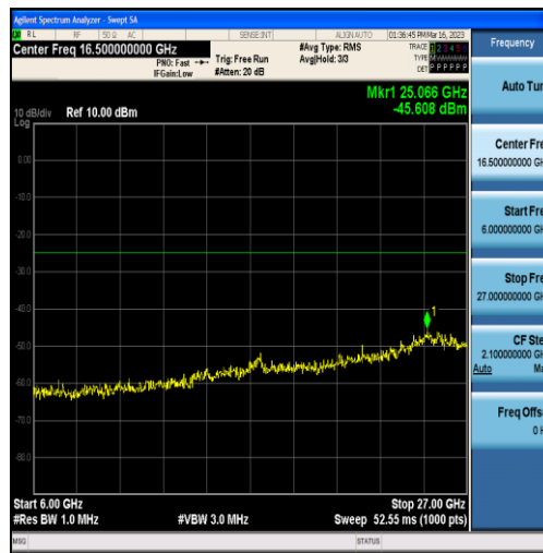
Band7-5MHz-QPSK-21100-25RB#0-Range3:6000~27000MHz
