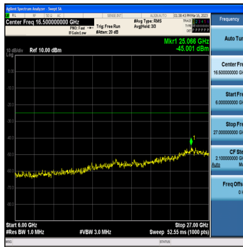
Band7-5MHz-QPSK-21425-25RB#0-Range3:6000~27000MHz
