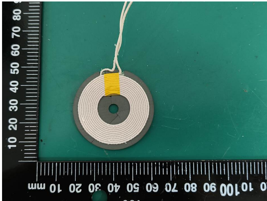
WPT ANT
