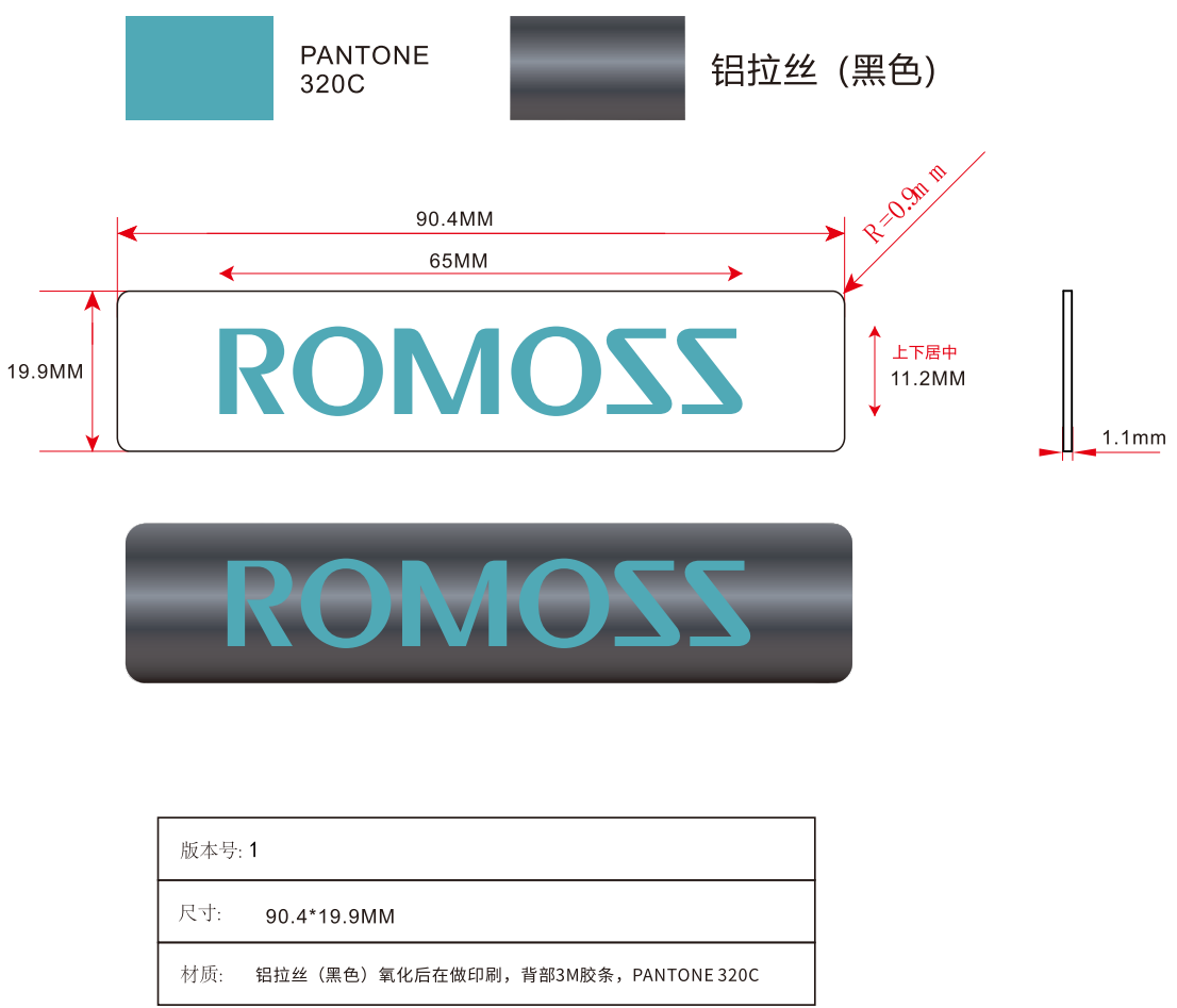
名称：铭牌
