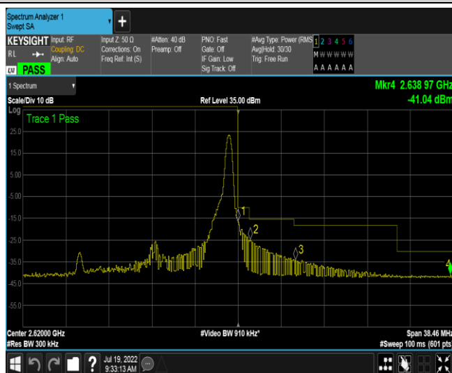
Band38-15MHz-QPSK-38175-1RB#74
