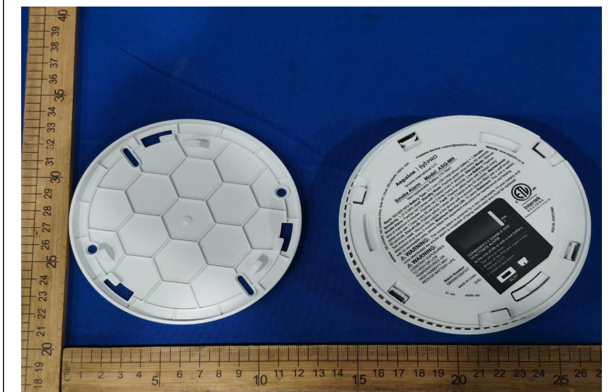
EUT Photo (14)
