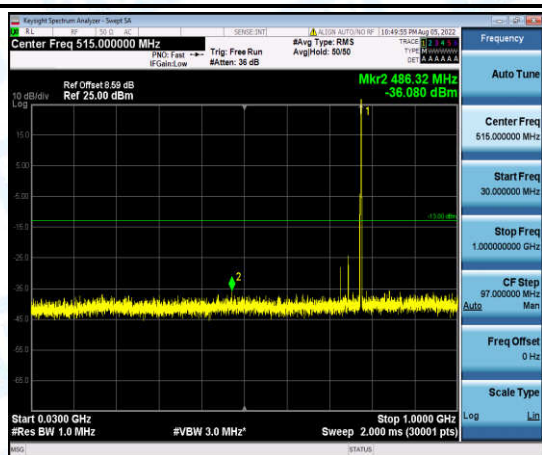
Band13-5MHz-QPSK-23230-1-0-Low-30-1000--36.08-PASS
