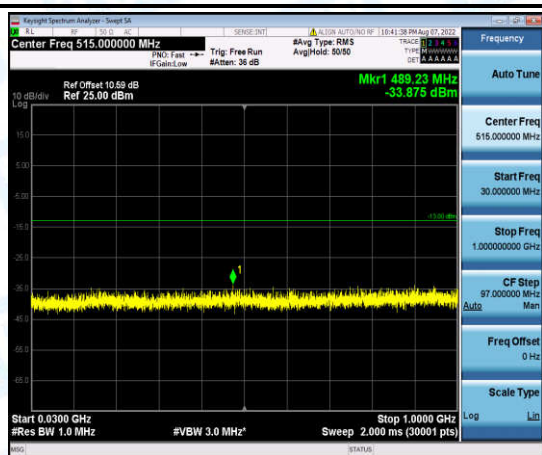
Band2-1.4MHz-QPSK-18900-1-0-Low-30-1000--33.88-PASS
