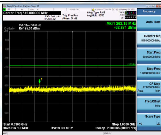
Band2-3MHz-QPSK-18900-1-0-Low-30-1000--32.87-PASS
