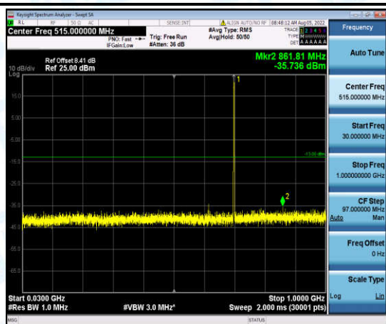
Band12-5MHz-QPSK-23095-1-0-Low-30-1000--35.74-PASS
