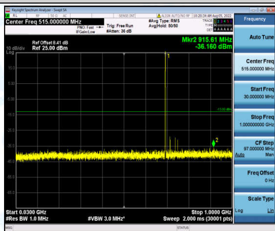
Band12-10MHz-QPSK-23060-1-0-Low-30-1000--36.16-PASS
