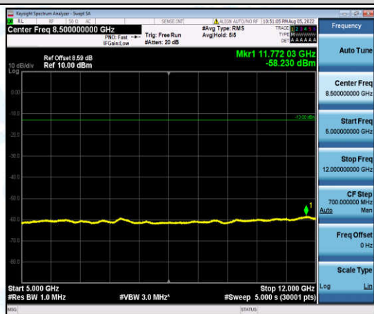
Band13-5MHz-QPSK-23230-1-0-Low-5000-12000--58.23-PASS
