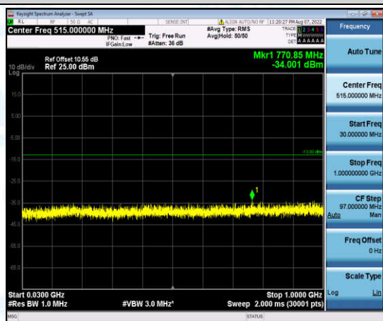
Band2-3MHz-16QAM-18615-1-0-Low-30-1000--34-PASS
