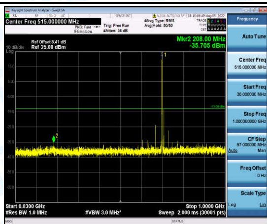
Band12-3MHz-16QAM-23095-1-0-Low-30-1000--35.71-PASS
