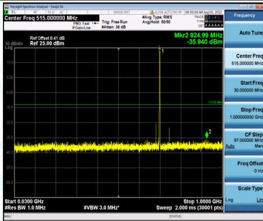
Band12-5MHz-16QAM-23095-1-0-Low-30-1000--35.94-PASS
