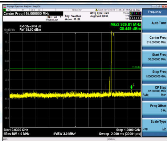
Band13-5MHz-16QAM-23230-1-0-Low-30-1000--35.45-PASS
