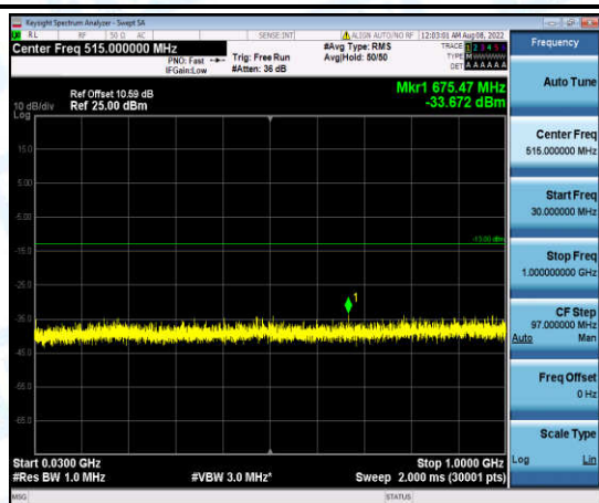
Band2-5MHz-QPSK-18900-1-0-Low-30-1000--33.67-PASS
