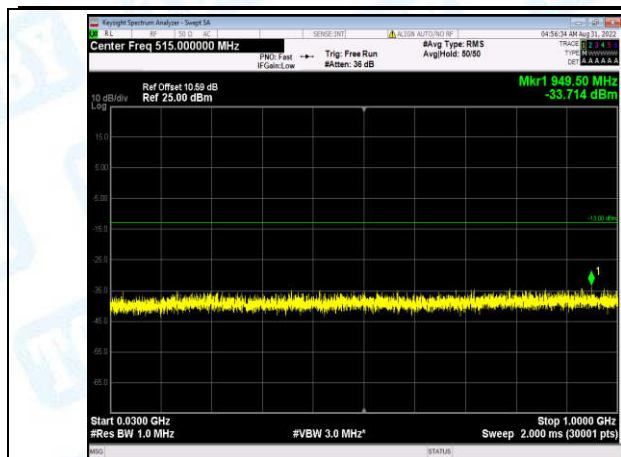
Band2-20MHz-QPSK-18900-1-0-Low-30-1000--33.71-PASS
