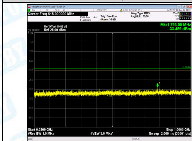
Band2-20MHz-QPSK-18700-1-0-Low-30-1000--33.46-PASS
