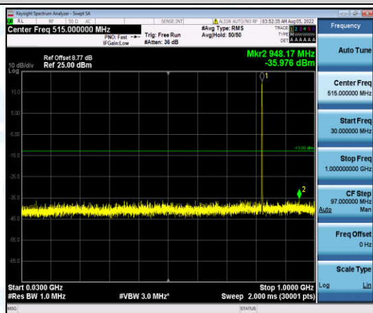
Band5-3MHz-QPSK-20415-1-0-Low-30-1000--35.98-PASS
