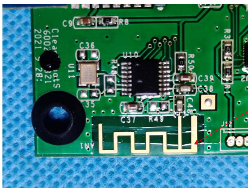
2.4G -RXAntenna
