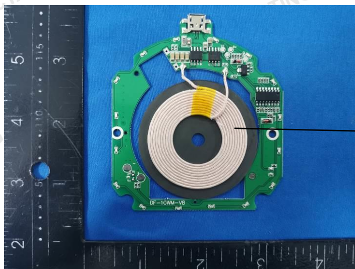
Antenna
