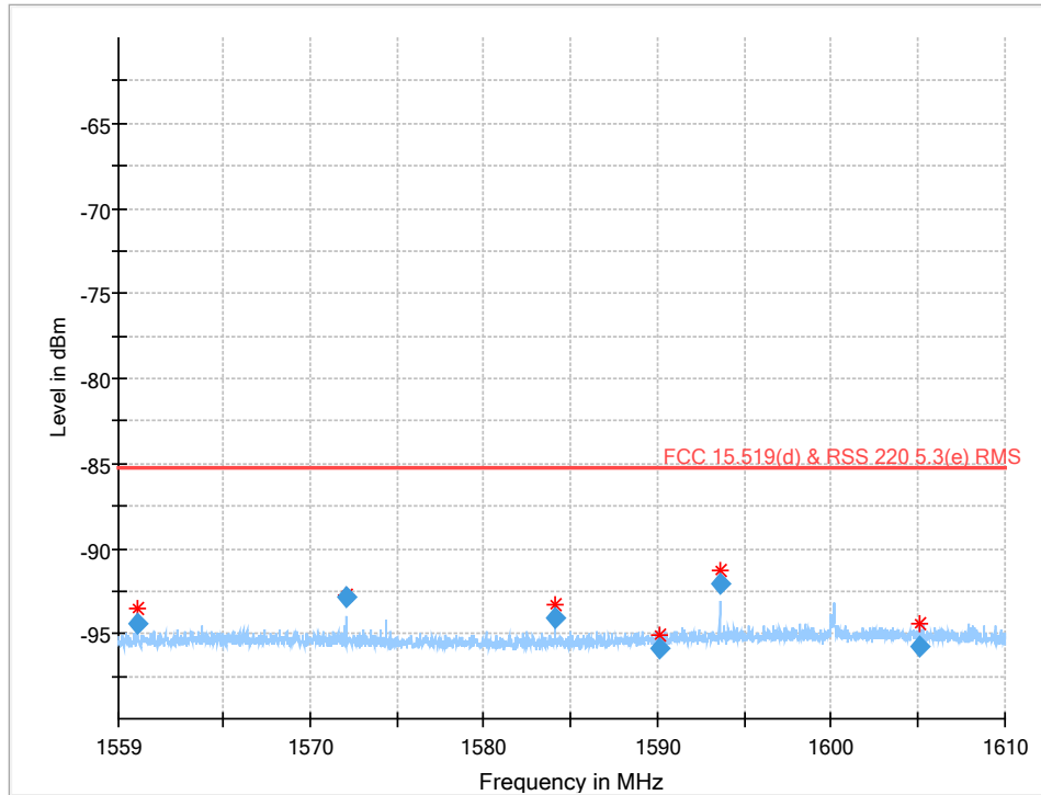
Plot 13: 1559 MHz to 1610 MHz (§15.519 (d), RSS-220 5.3.1(e)) (EUT2)
