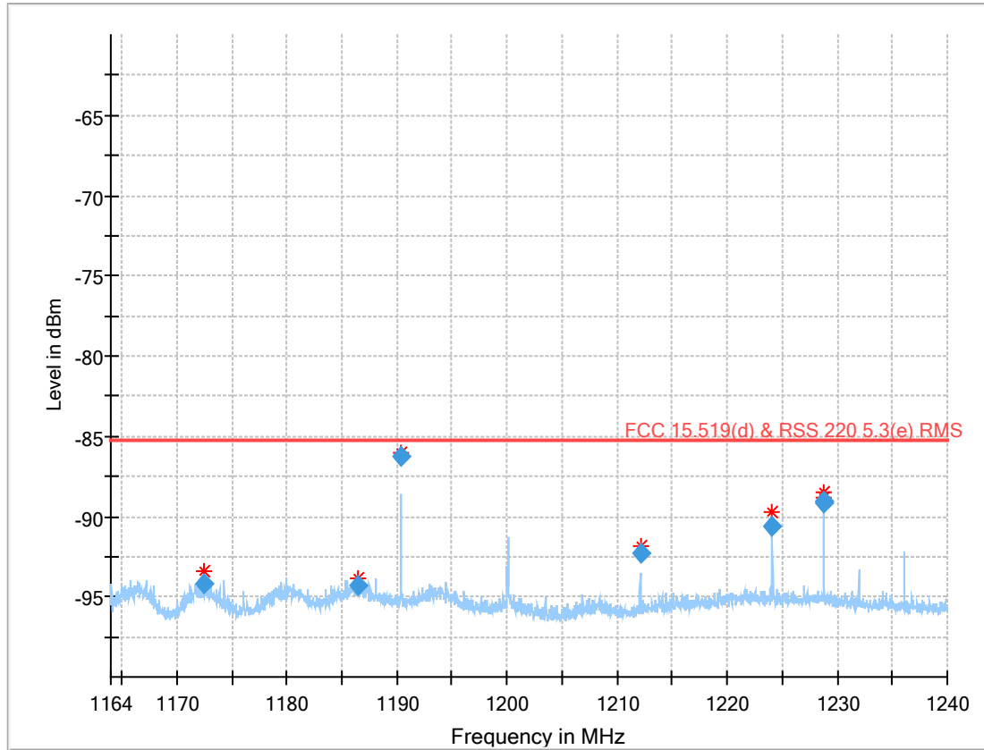
Plot 12: 1164 MHz to 1240 MHz (§15.519 (d), RSS-220 5.3.1(e)) (EUT2)
