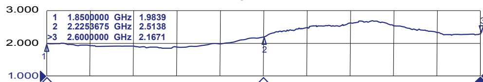
VSWR
