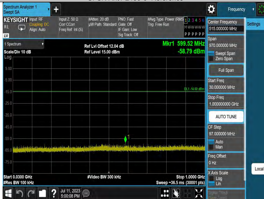
GFSK-Ant1-2480-30~1000
