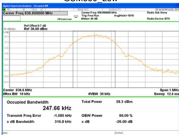
GSM850_Middle
