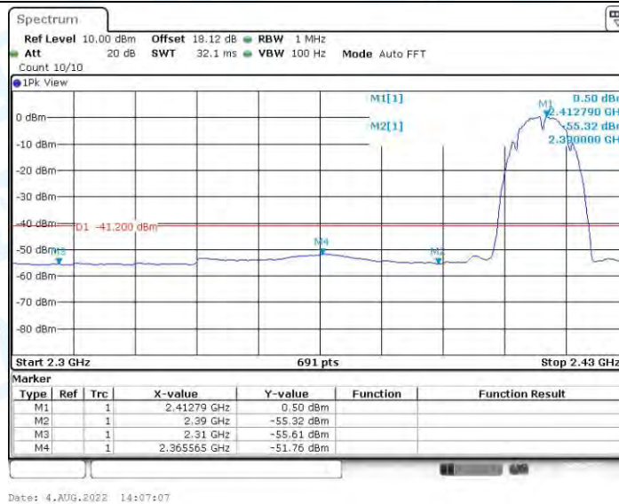
11B-CDD_Ant1_Low_2412_AV
