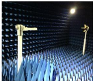
ETS 暗室
