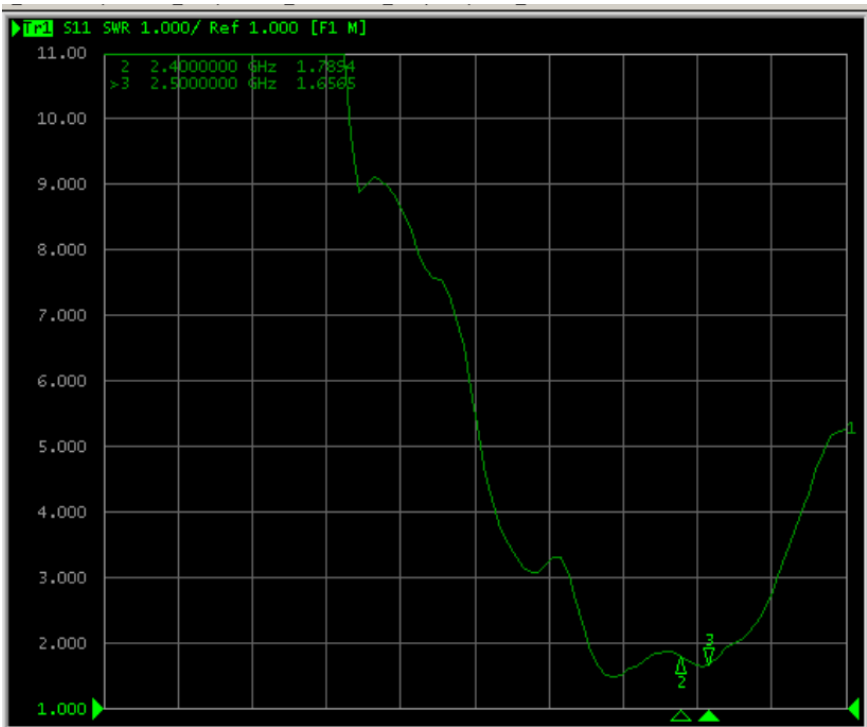
VSWR
