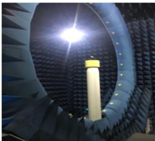
SATIMO 暗室
