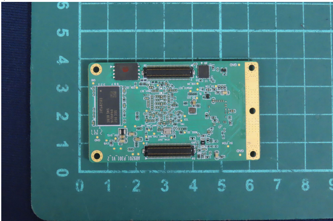
(2) EUT Photo
