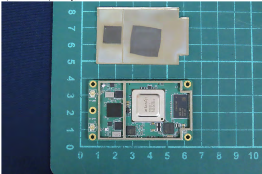
(16) EUT Photo (RF Chip)
