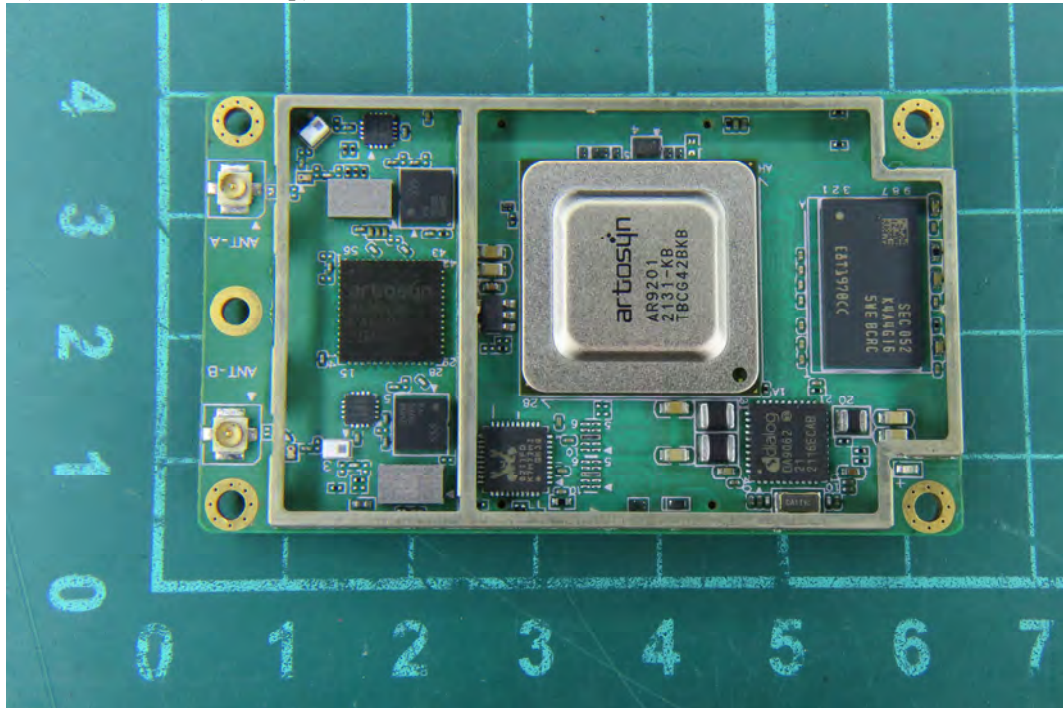
(17) EUT Photo (RF Chip)
