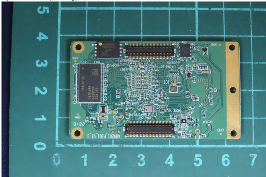
(18) EUT Photo (RF Chip)
