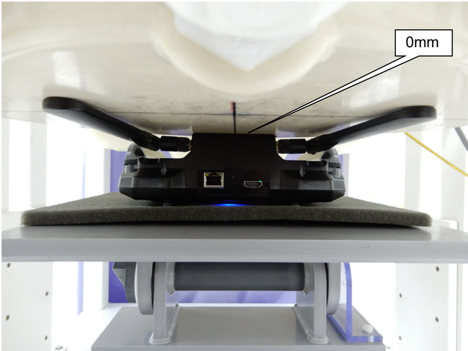
EUT Back_0mm
