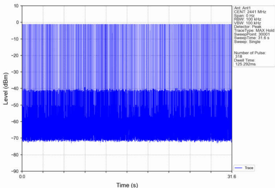
Pi/4DQPSK_2DH1_HOPP_Ant1_NTNV
