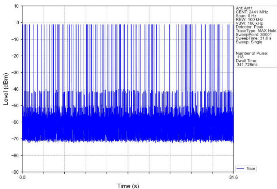
Pi/4DQPSK_2DH5_HOPP_Ant1_NTNV
