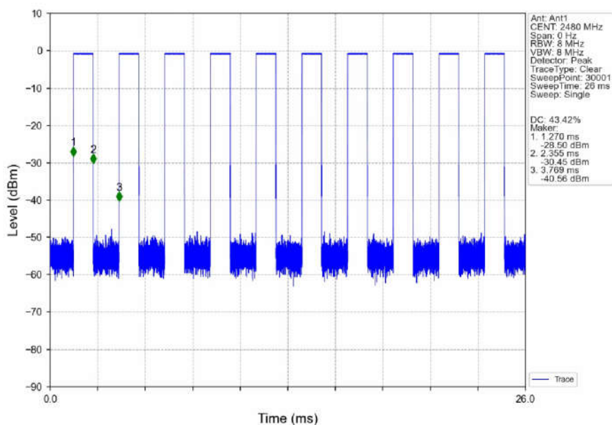
2M_HCH_2480MHz_Ant1_NTNV
