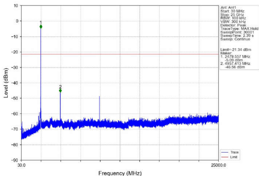
2M_HCH_2480MHz_Ant1_NTNV
