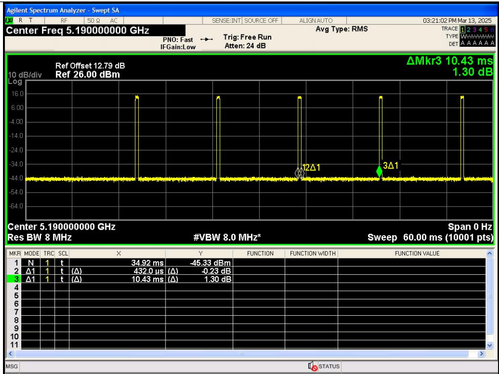
IEEE 802.11ac_40MHz_Channel 38
