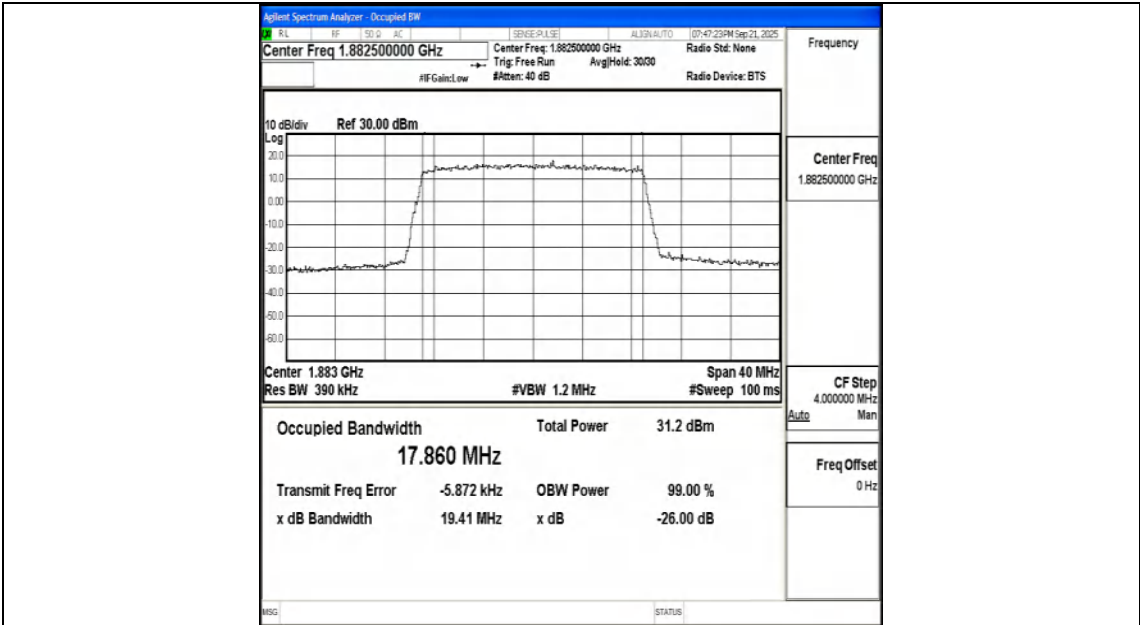
Band25-20MHz-QPSK-26365-100RB#0-PASS
