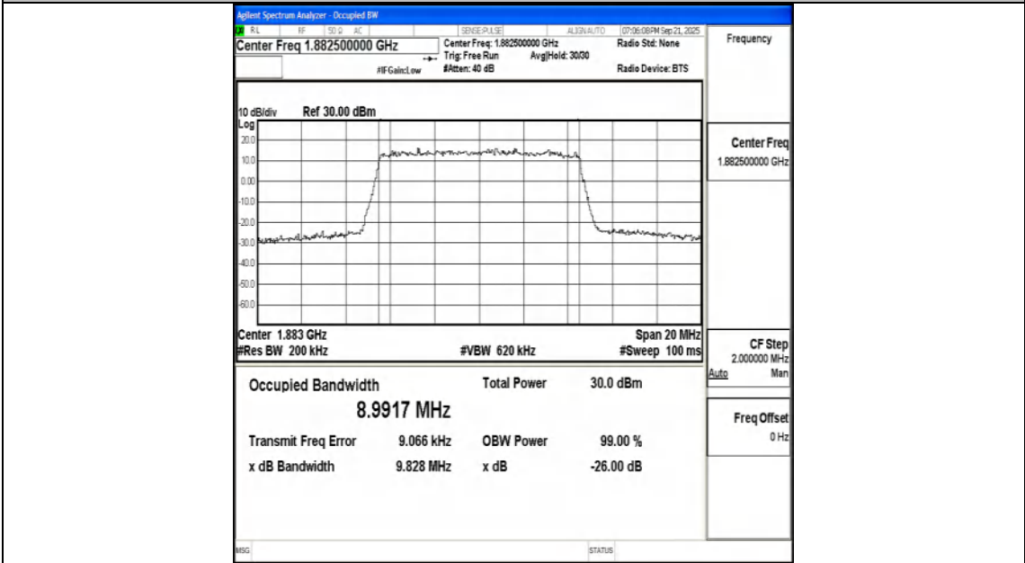
Band25-10MHz-16QAM-26365-50RB#0-PASS
