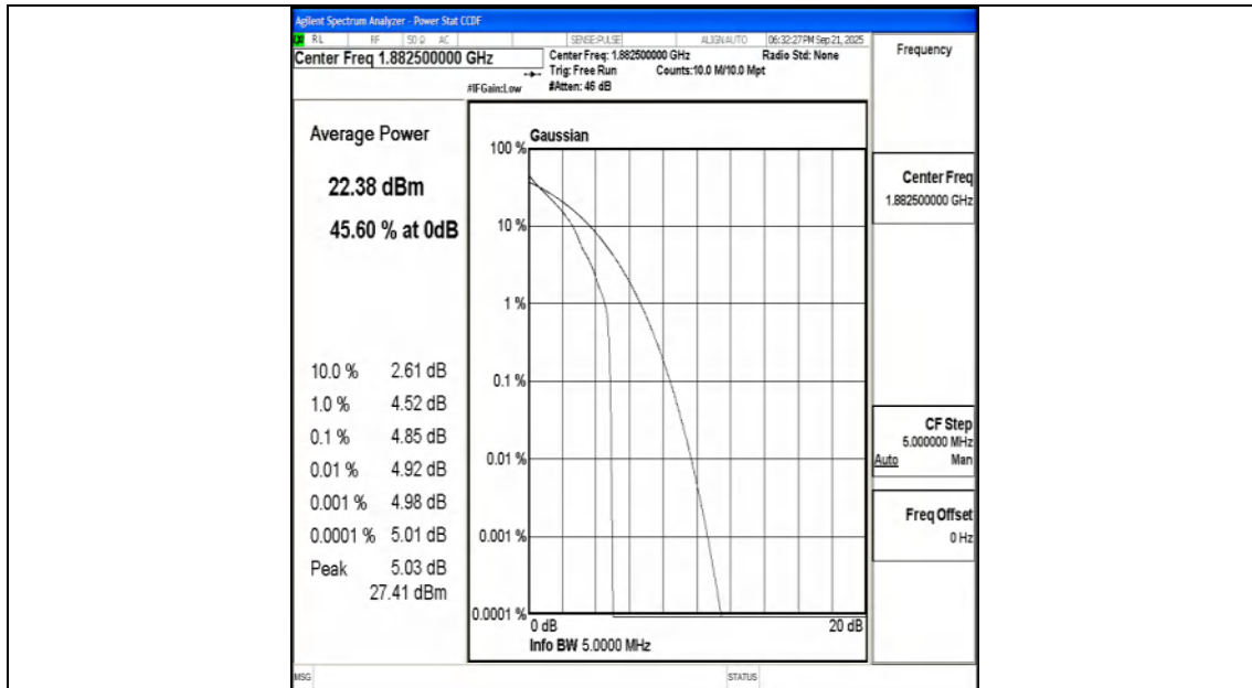
Band25-3MHz-QPSK-26365-1RB#0-PASS
