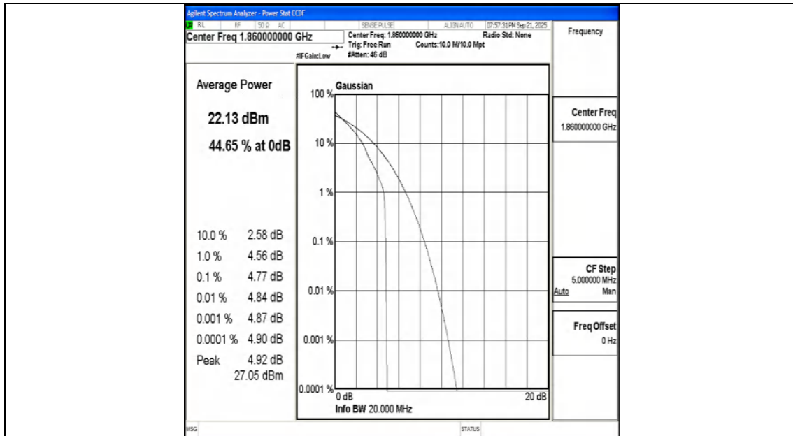
Band25-20MHz-QPSK-26140-1RB#0-PASS
