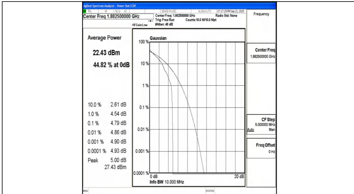
Band25-10MHz-QPSK-26365-1RB#0-PASS
