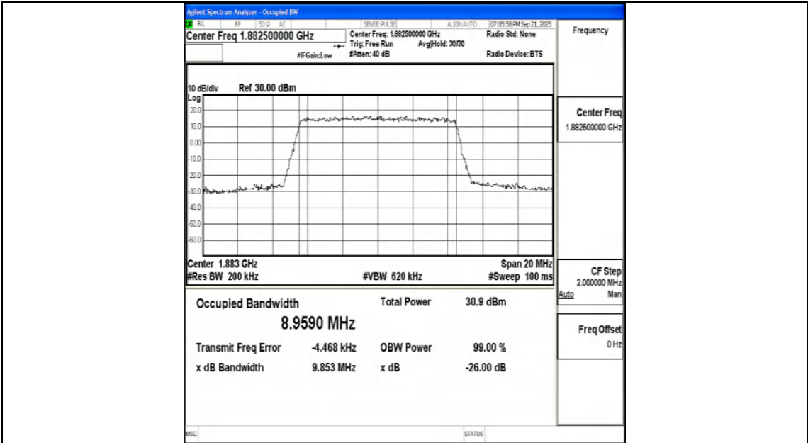
Band25-10MHz-QPSK-26365-50RB#0-PASS
