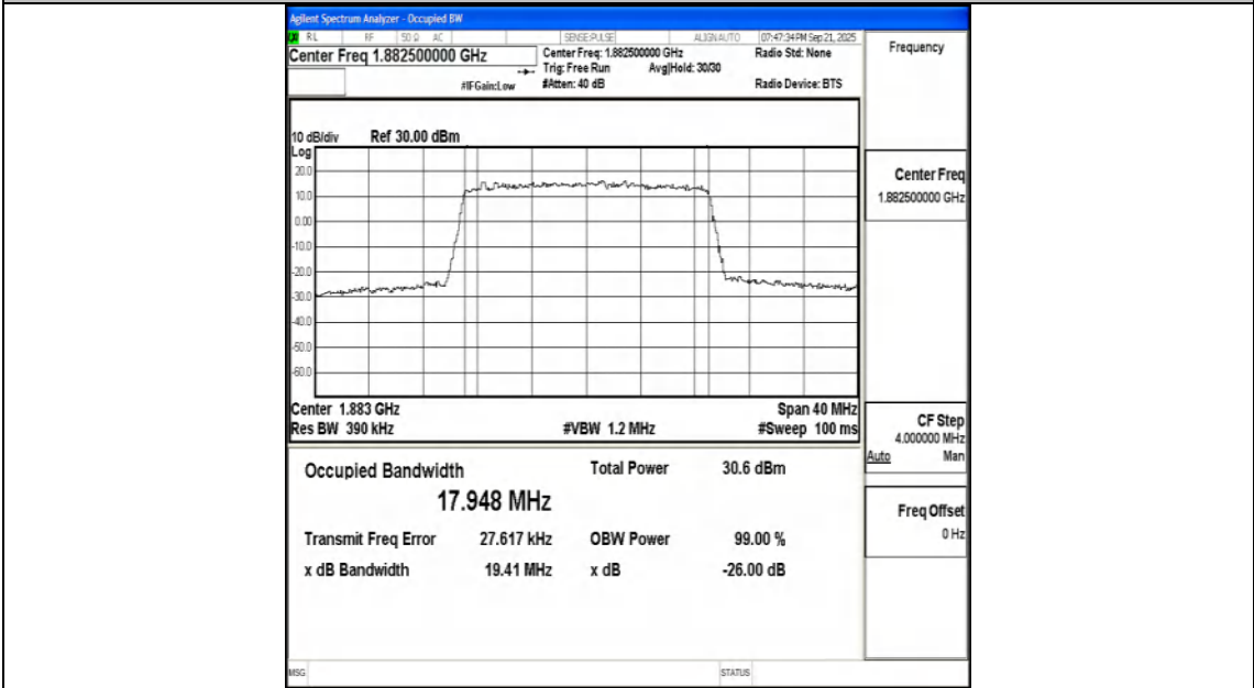
Band25-20MHz-16QAM-26365-100RB#0-PASS
