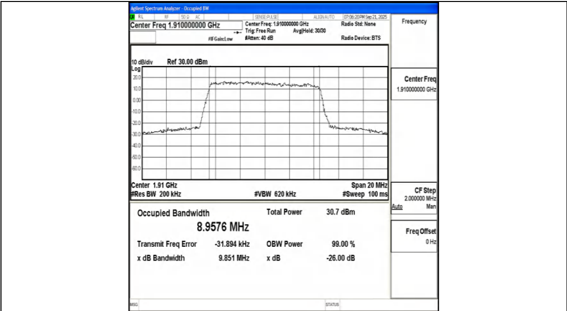
Band25-10MHz-QPSK-26640-50RB#0-PASS
