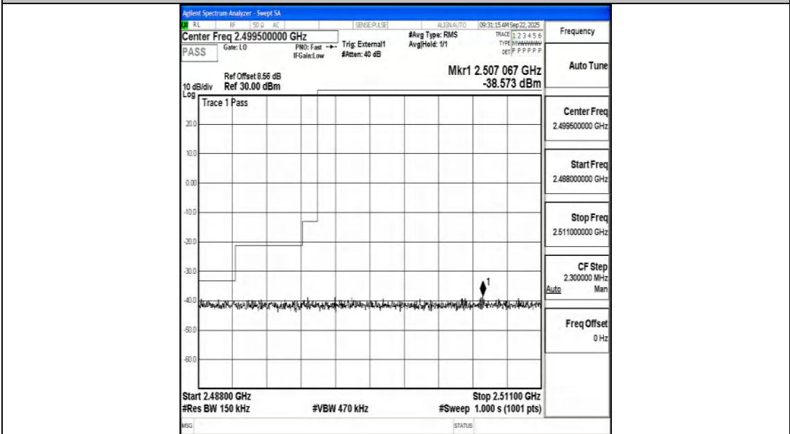
Band41_15MHz_QPSK_39725_75RB#0
