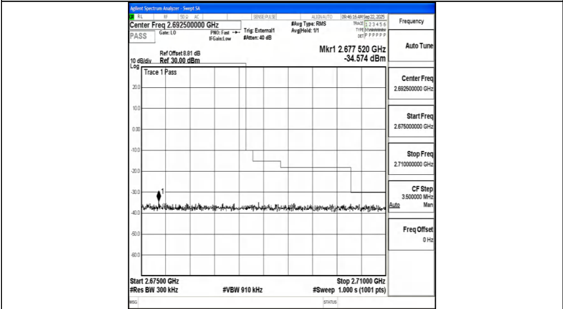
Band41_15MHz_QPSK_41515_75RB#0
