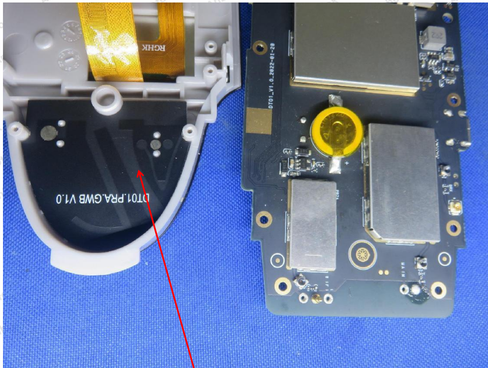
BT/WIFI/GPS(RX) ANT
