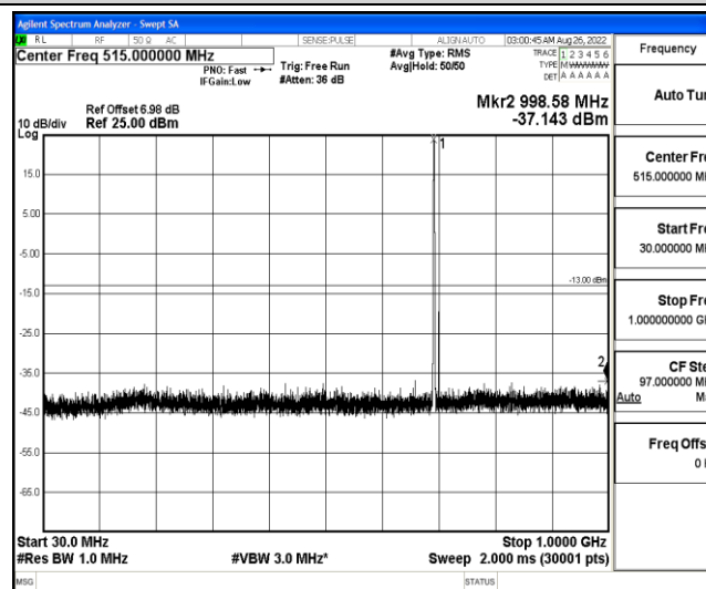
Band12-3MHz-QPSK-23025-1-0-Low-30-1000--37.14-PASS
