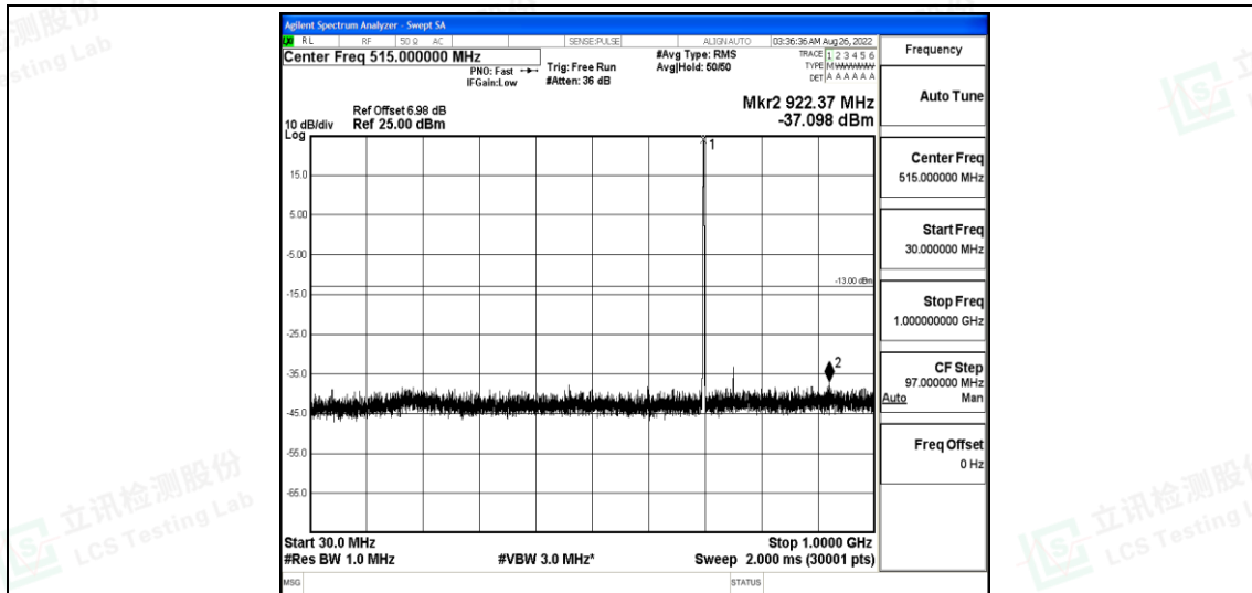
Band12-5MHz-16QAM-23095-1-0-Low-30-1000--37.1-PASS
