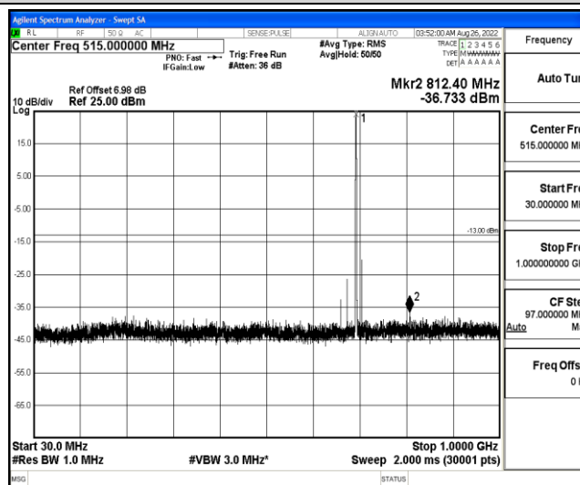
Band12-10MHz-QPSK-23060-1-0-Low-30-1000--36.73-PASS
