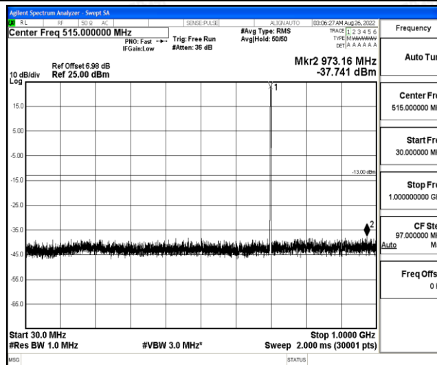
Band12-3MHz-16QAM-23095-1-0-Low-30-1000--37.74-PASS
