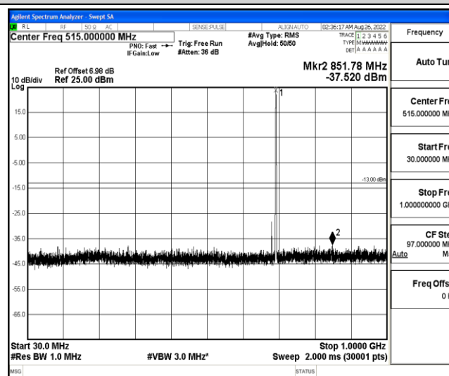
Band12-1.4MHz-16QAM-23017-1-0-Low-30-1000--37.52-PASS
