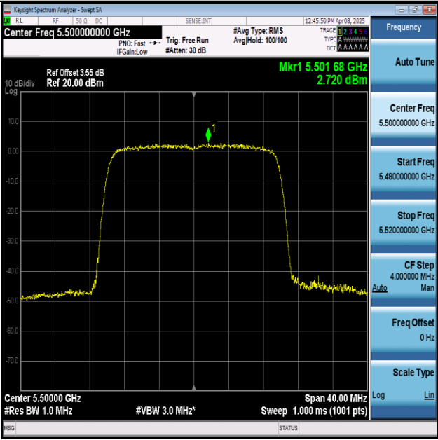
11AX20MIMO-Ant1-5500-PASS
