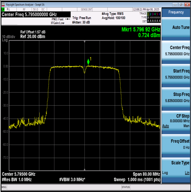
11N40MIMO-Ant1-5795-PASS
