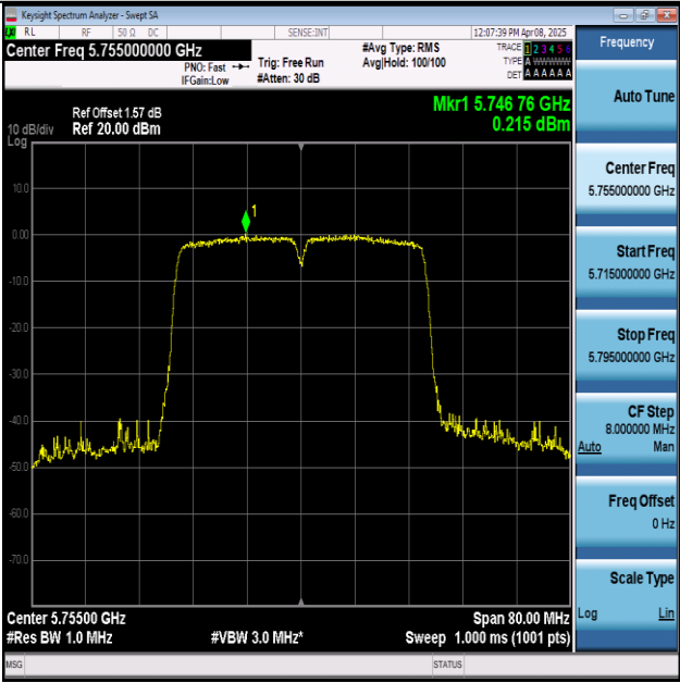
11N40MIMO-Ant1-5755-PASS
