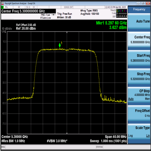
11AX20MIMO-Ant1-5300-PASS
