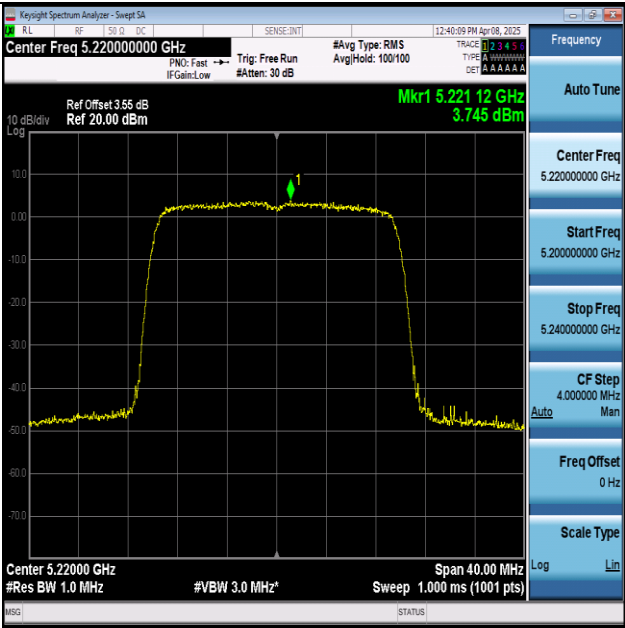
11AX20MIMO-Ant1-5220-PASS
