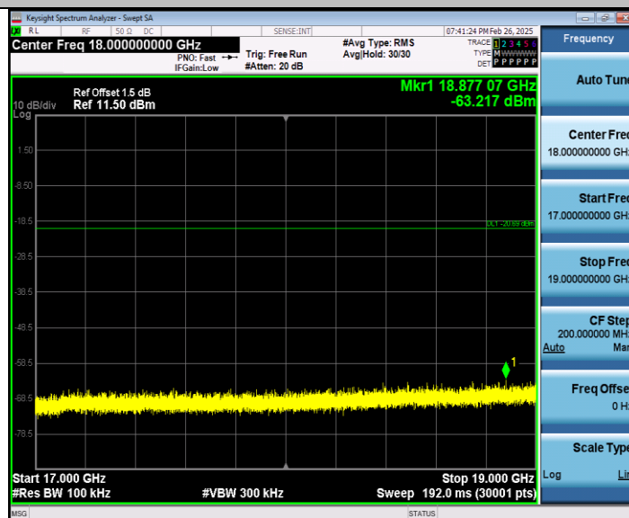
2DH5_Ant1_2402_19000~21000
