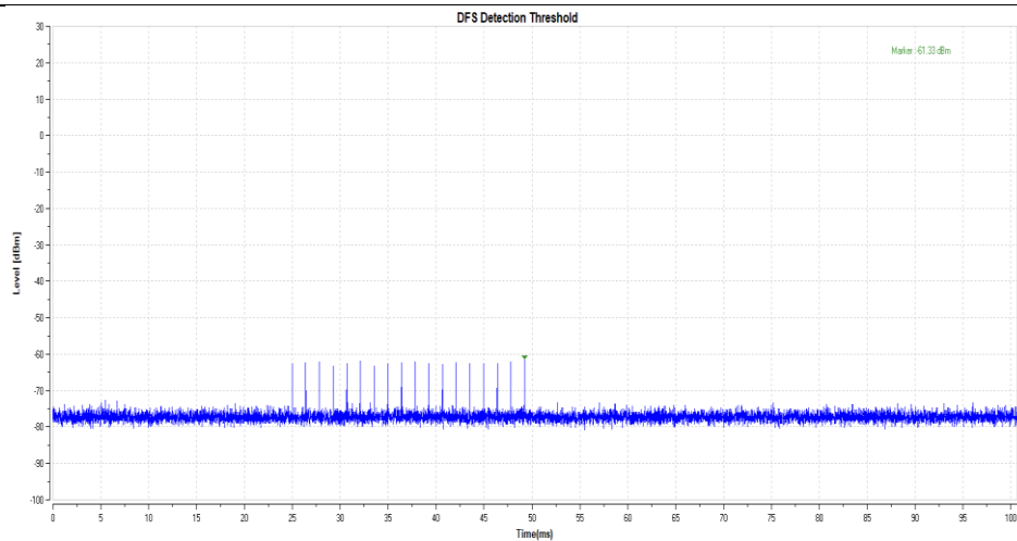
11A-5260-Type0
