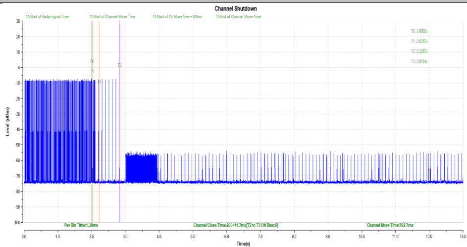
11A-5500-Type0
