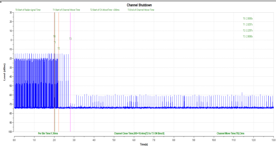
11AC80SISO-5290-Type0
