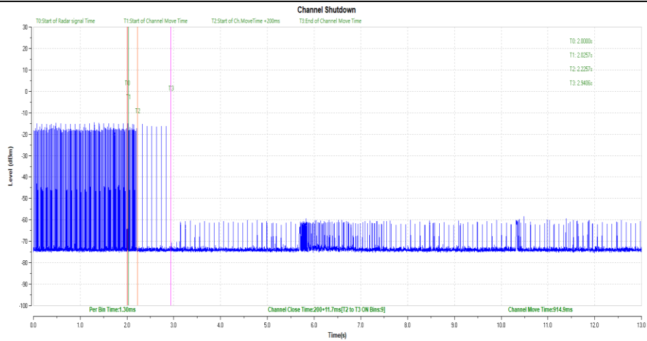
11N40SISO-5270-Type0
