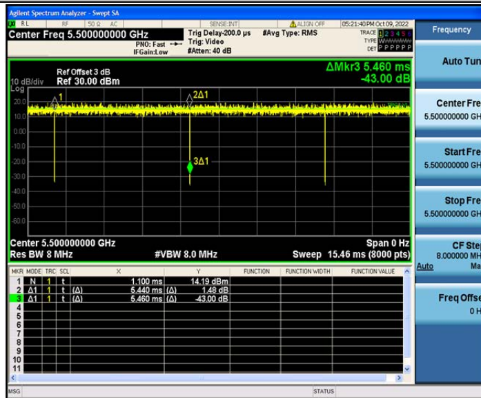
802.11ax(HE20)_Ant2_5500
