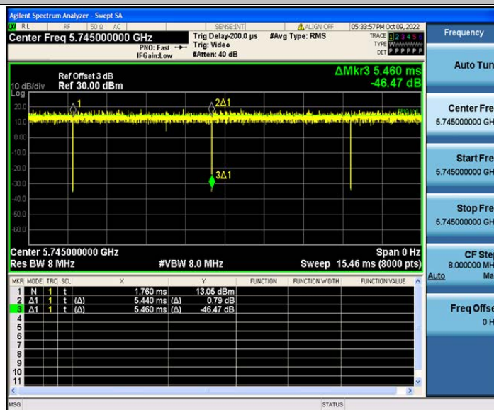
802.11ax(HE20)_Ant2_5745
