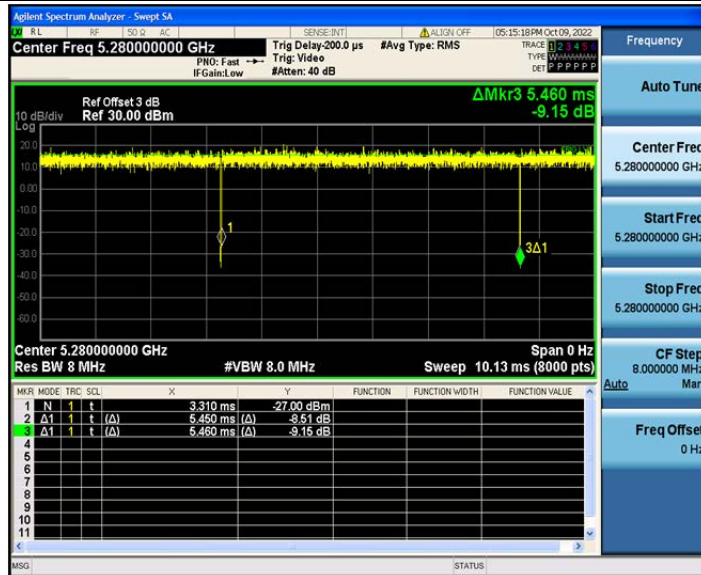
802.11ax(HE20)_Ant2_5280
