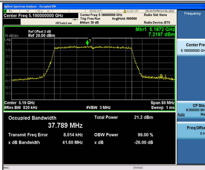
802.11ax(HE40)_Ant2_5190 484/65
