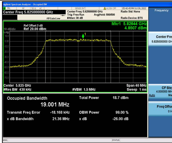
802.11ax(HE20)_Ant2_5825 242/61
