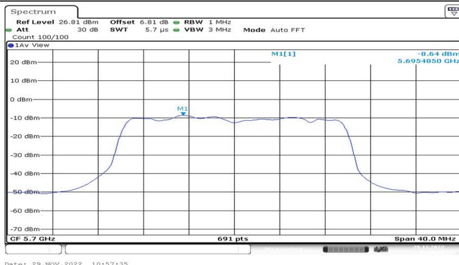
802.11ax(HE20)_Ant2_5700 52/38
