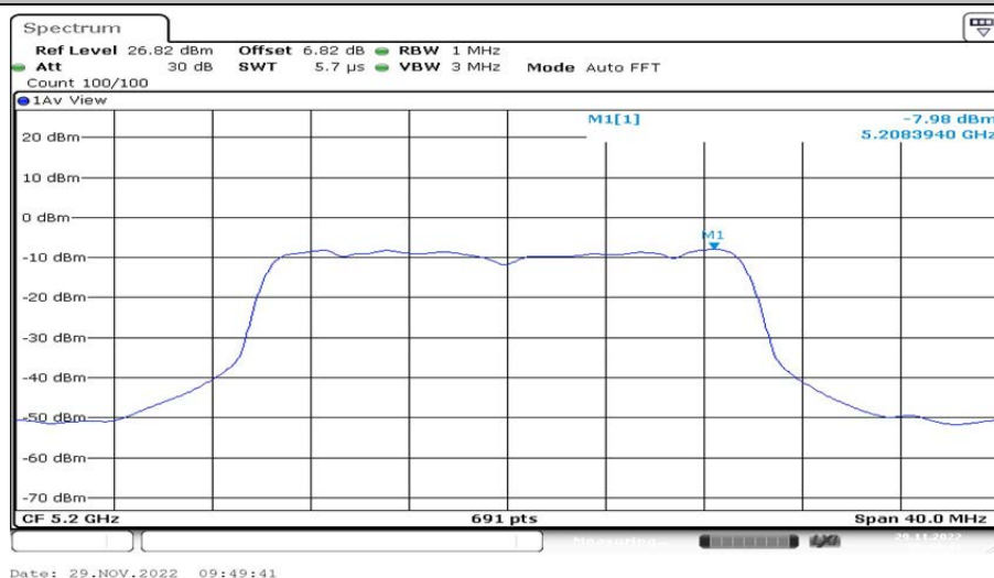
802.11ax(HE20)_Ant2_5200 52/38
