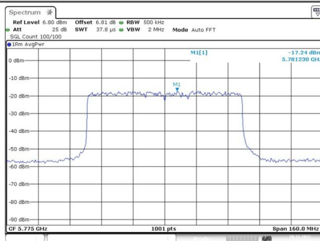
802.11ax(HE80)_Ant1_5775 26/19
