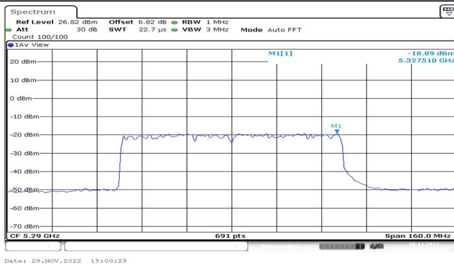
802.11ax(HE80)_Ant2_5290 242/62
