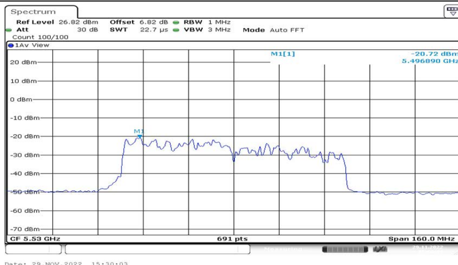
802.11ax(HE80)_Ant2_5530 242/62
