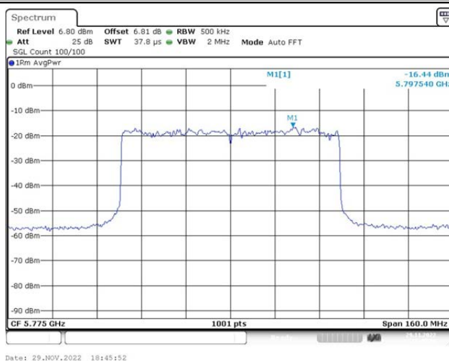
802.11ax(HE80)_Ant2_5775 242/62
