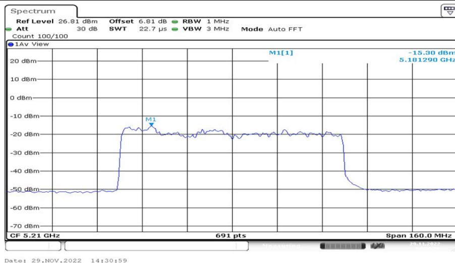
802.11ax(HE80)_Ant2_5210 242/62
