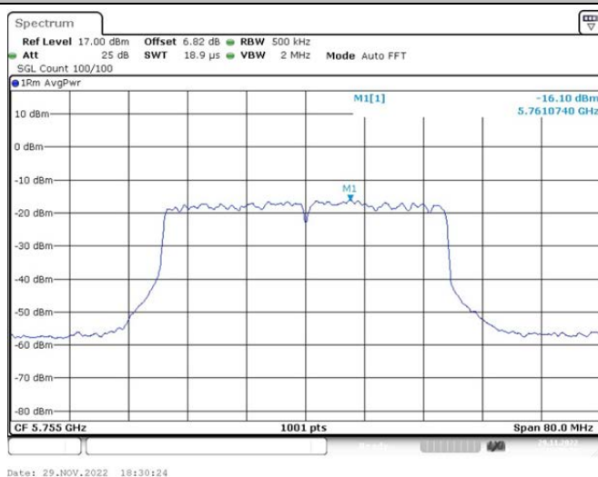
802.11ax(HE40)_Ant2_5755 242/61
