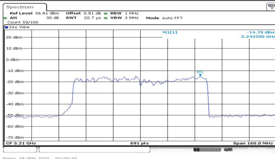
802.11ax(HE80)_Ant2_5210 52/44
