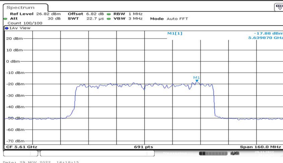
802.11ax(HE80)_Ant2_5610 242/62
