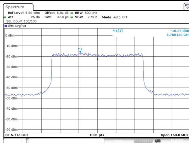
802.11ax(HE80)_Ant1_5775 484/65
