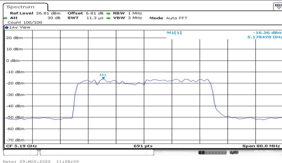
802.11ax(HE40)_Ant2_5190 242/61
