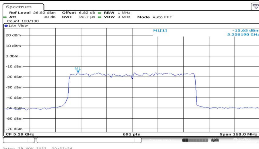
802.11ax(HE80)_Ant2_5290 52/44
