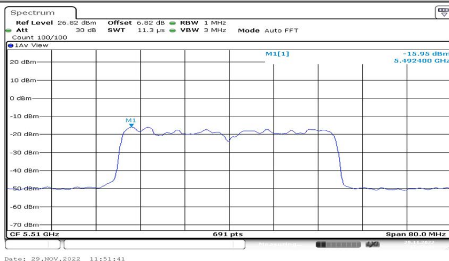
802.11ax(HE40)_Ant2_5510 242/61
