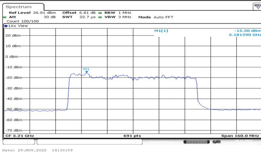
802.11ax(HE80)_Ant2_5210 106/56
