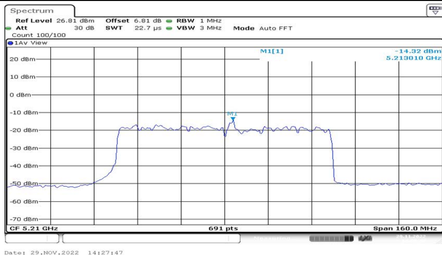
802.11ax(HE80)_Ant2_5210 26/19
