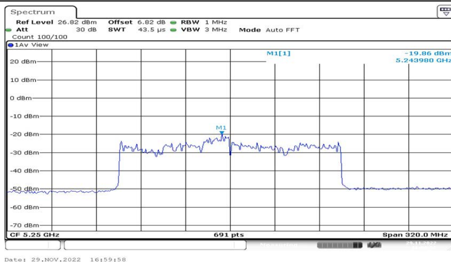
802.11ax(HE160)_Ant2_5250 242/64
