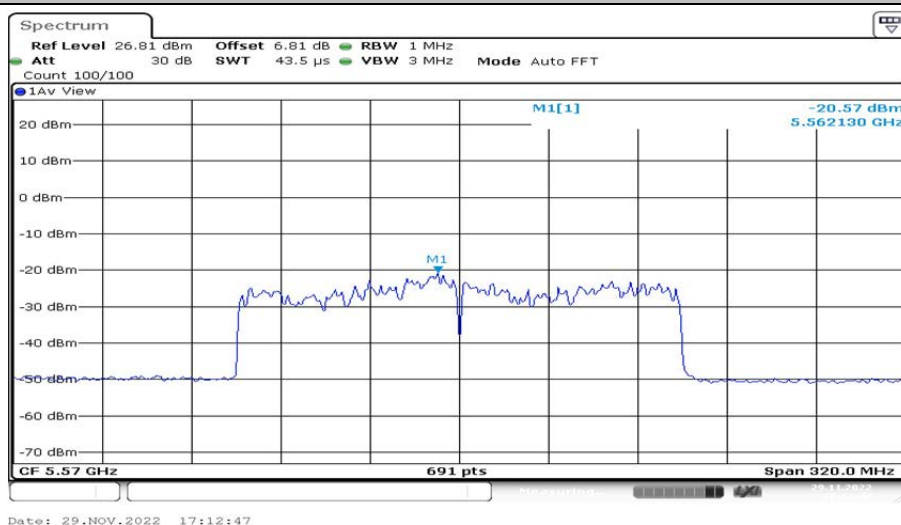
802.11ax(HE160)_Ant2_5570 242/64
