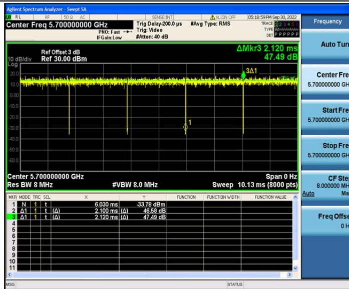
802.11a_Ant2_5700
