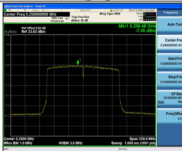
802.11ax(HE160)_Ant2_5250 996*2/68
