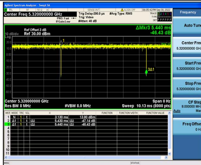
802.11n(HT20)_Ant2_5320
