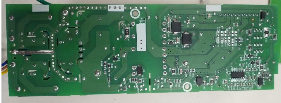
IP extension board ICIP30
