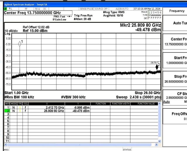
11B_Ant1_2412_1000~26500
