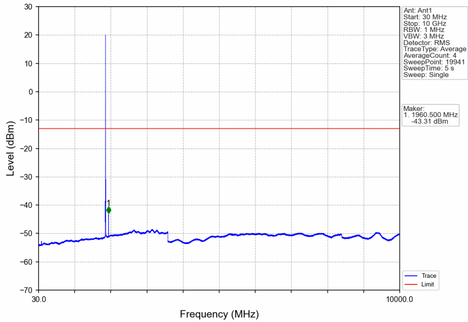
Band2_3MHz_QPSK_MCH_1880MHz_RB_1_0_NTNV
