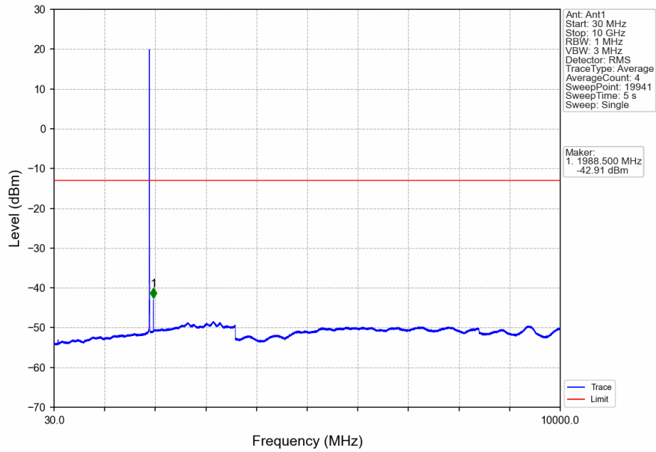
Band2_3MHz_QPSK_HCH_1908.5MHz_RB_1_0_NTNV
