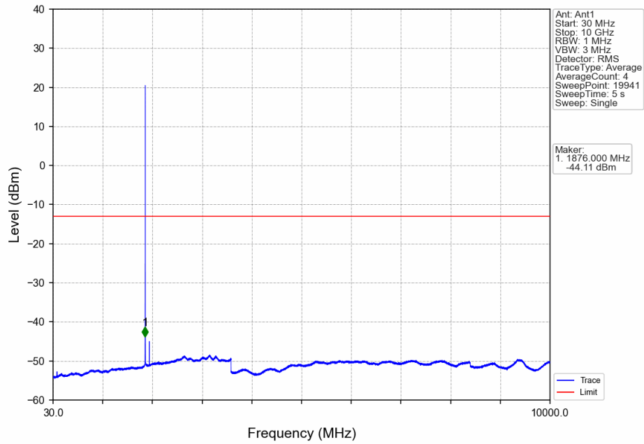
Band2_1.4MHz_QPSK_MCH_1880MHz_RB_1_0_NTNV
