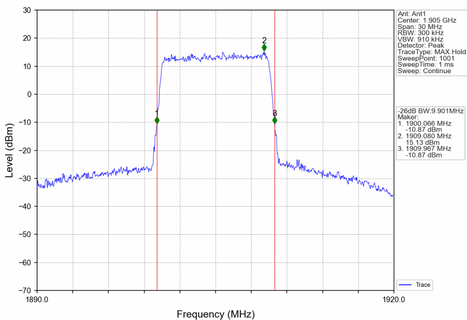
Band2_10MHz_16QAM_HCH_1905MHz_RB_50_0_NTNV
