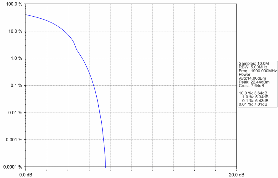
Band2_20MHz_QPSK_HCH_1900MHz_RB_100_0_NTNV
