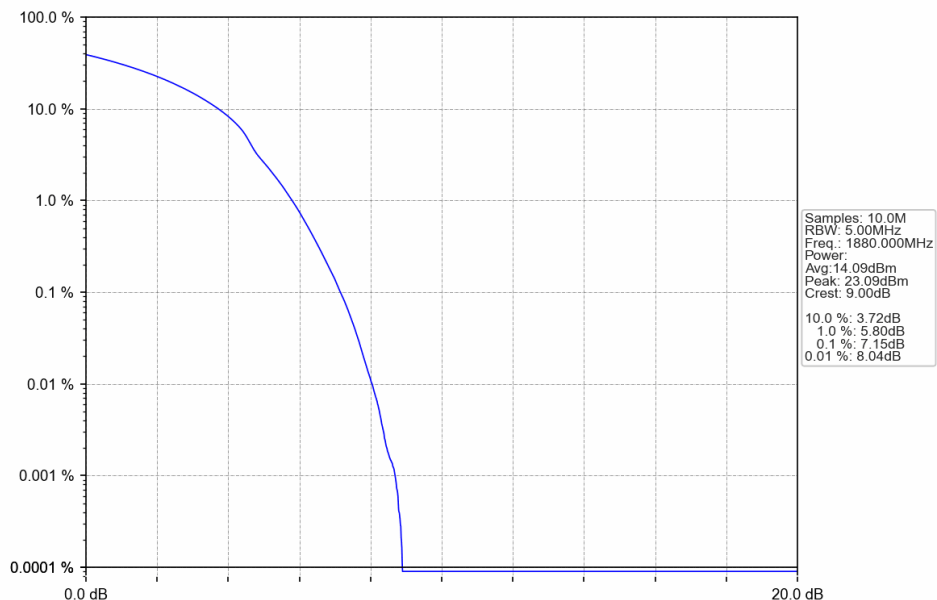
Band2_20MHz_16QAM_MCH_1880MHz_RB_100_0_NTNV
