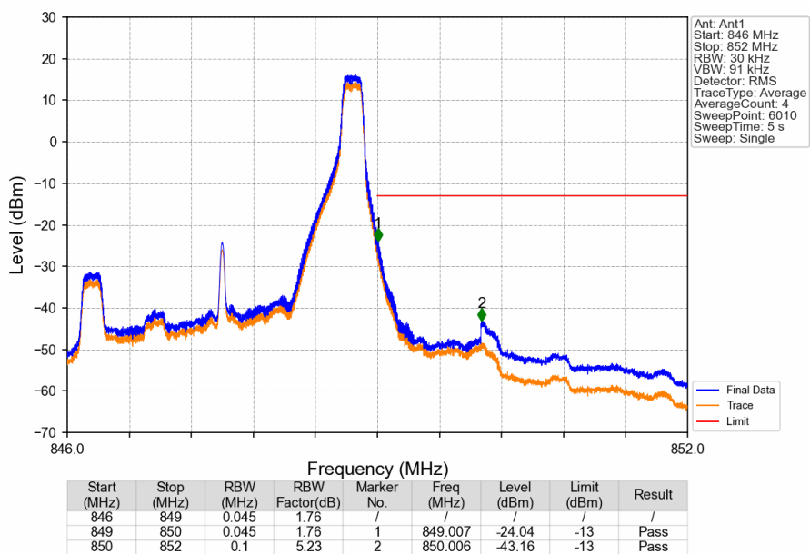
Band5_3MHz_QPSK_HCH_847.5MHz_RB_1_14_NTNV
