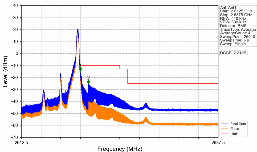
Band38_5MHz_QPSK_HCH_2617.5MHz_RB_1_24_NTNV
