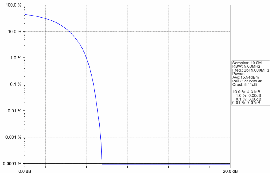
Band38_10MHz_QPSK_HCH_2615MHz_RB_50_0_NTNV
