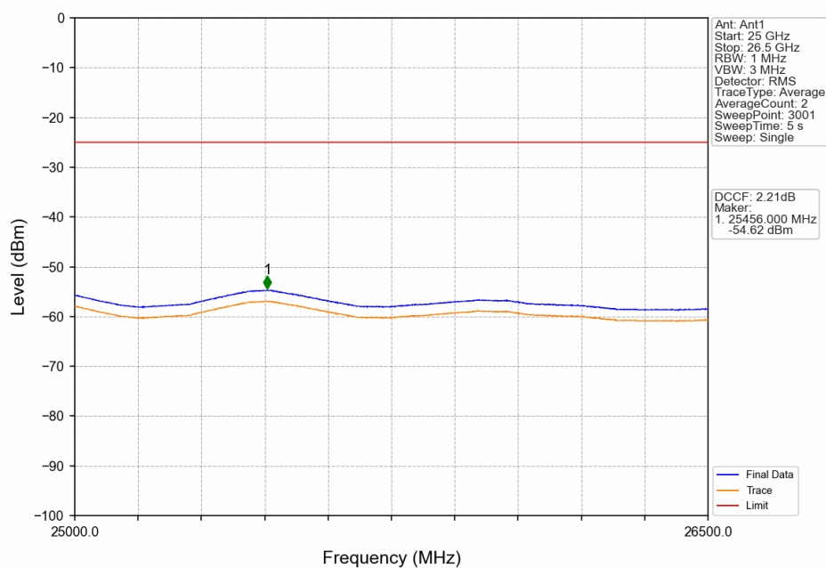
Band38_5MHz_QPSK_LCH_2572.5MHz_RB_1_0_NTNV
