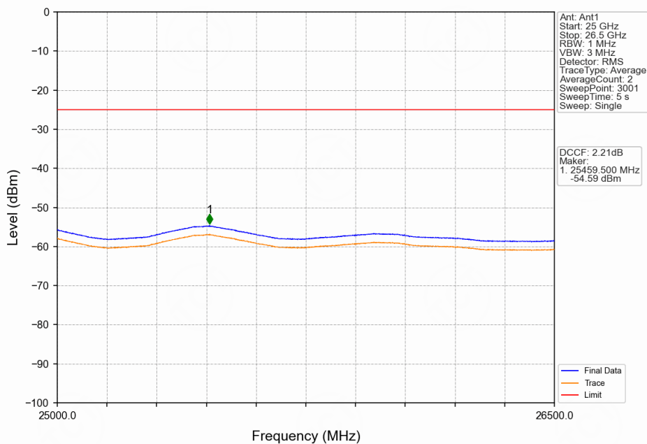
Band38_5MHz_QPSK_HCH_2617.5MHz_RB_1_24_NTNV
