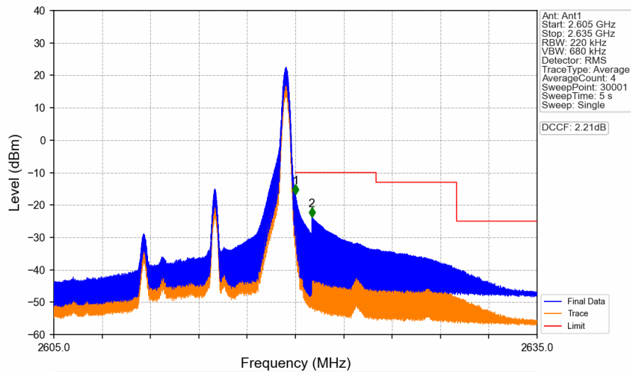
Band38_10MHz_QPSK_HCH_2615MHz_RB_1_49_NTNV
