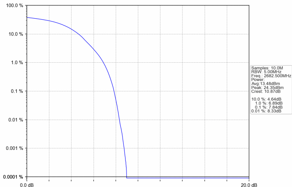
Band41_15MHz_QPSK_HCH_2682.5MHz_RB_75_0_NTNV
