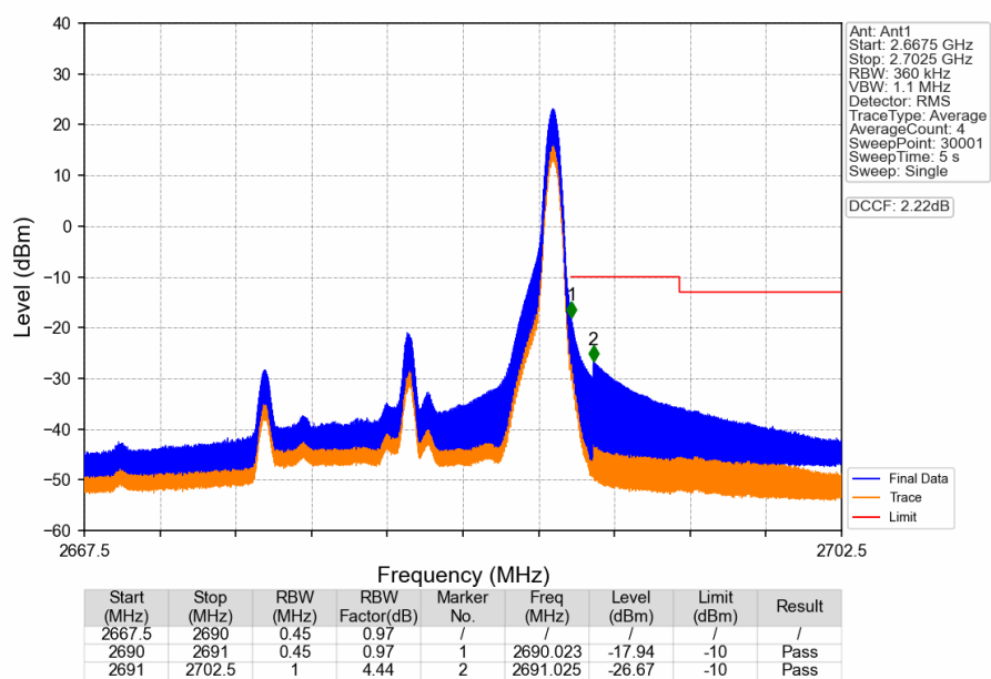
Band41_15MHz_QPSK_HCH_2682.5MHz_RB_1_74_NTNV
