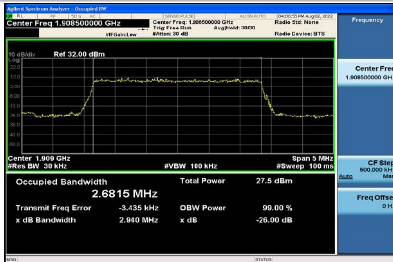
Band2-3MHz-QPSK-19185-15RB#0-2.6815
