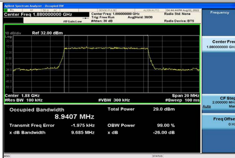
Band2-10MHz-QPSK-18900-50RB#0-8.9407
