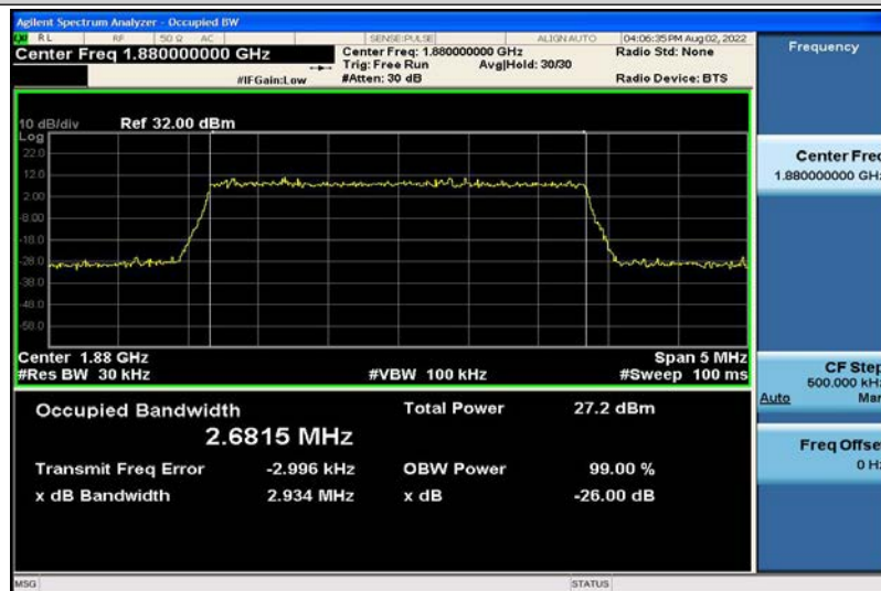
Band2-3MHz-QPSK-18900-15RB#0-2.6815
