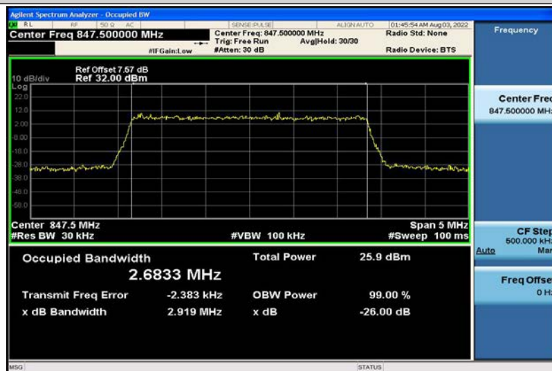
Band5-3MHz-QPSK-20635-15RB#0-2.6833
