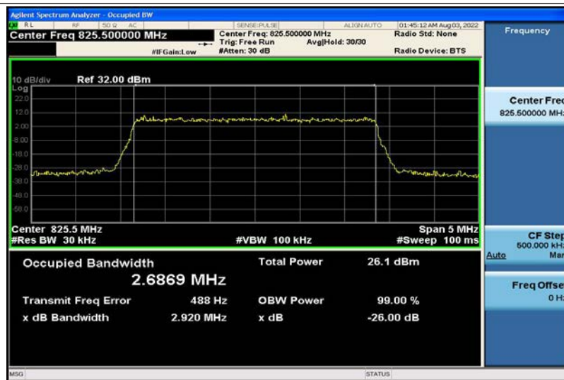
Band5-3MHz-QPSK-20415-15RB#0-2.6869
